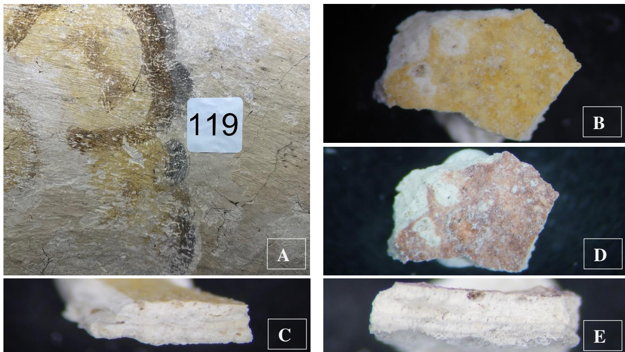
30 pav. Mėginys P18 – Zn-119 (geltona spalva (gėlė)): A – paėmimo vieta; B – mėginio vaizdas pro mikroskopą, x20; C – mėginio, skerspjūvio vaizdas pro mikroskopą, x 40; D – mėginio, iškaitinto 600 °C temperatūroje, vaizdas pro mikroskopą, x 40; E – mėginio, iškaitinto 600 °C temperatūroje, skerspjūvio vaizdas pro mikroskopą, x 40
