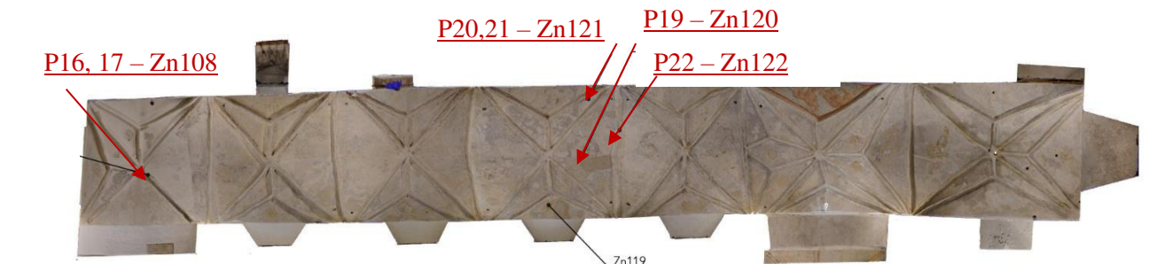
28 pav. Mėginių paėmimo vietos stratigrafiniams ir cheminiams polichrominio dekoru tyrimams
