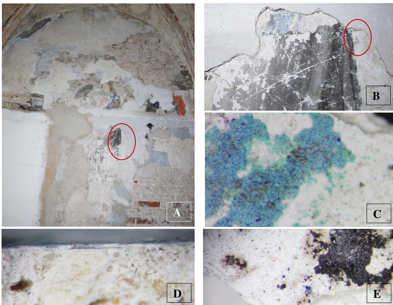
25 pav. Mėginys P14 (melsvai-žalsva): A, B – mėginio paėmimo vieta; C – mėginio vaizdas pro mikroskopą, 40; D – mėginio, skerspjūvio vaizdas pro mikroskopą, x 40; E – mėginio, iškaitinto 600 °C temperatūroje, vaizdas pro mikroskopą, x 40.
