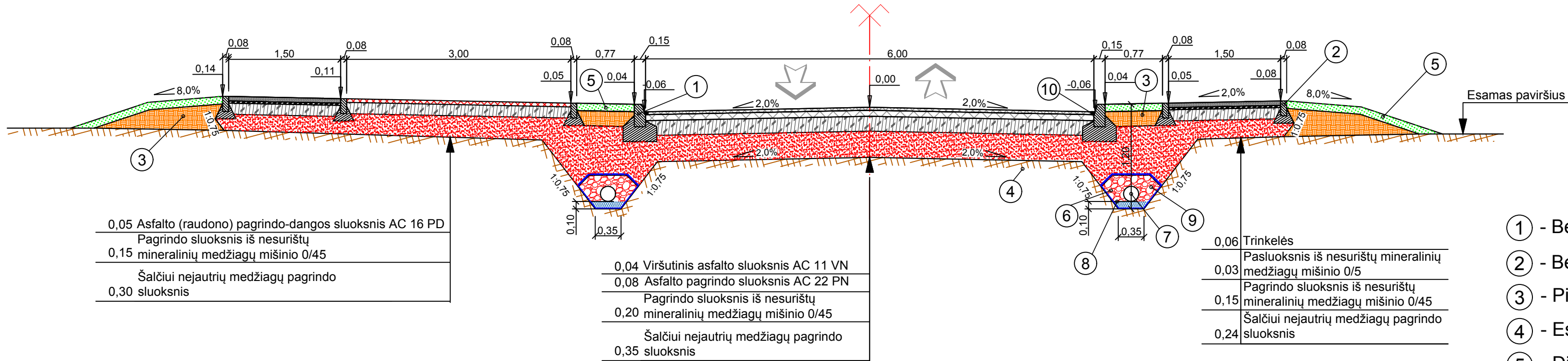
Debesų gatvės skersinis profilis Nr.1
