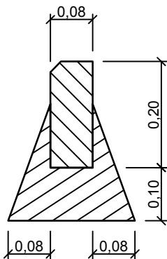
Vejos bordiūro detalė M 1:10
