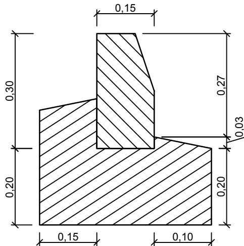
Gatvės bordiūro 100.30.15 detalė M 1:10
