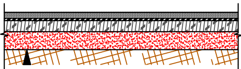
Skersinio profilio pjūvis per nuovažą M 1:50
