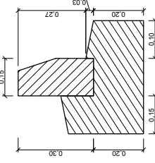
Vejos bordiūro detalē M 1:10
