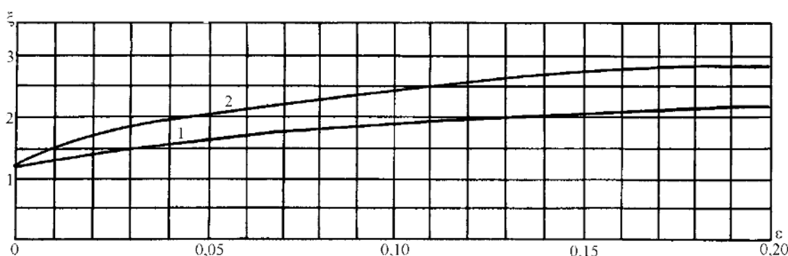
Pav. 9 Dinaminiai koeficientai: 1 – gelžbetoniniams ir mūro statiniams; 2 – plieniniams bokštams, stiebams, futeruotiems dūmtraukiams, kolonų tipo aparatams, įskaitant esančius ant gelžbetoninių paaukštinių ( d = 0,15 )
