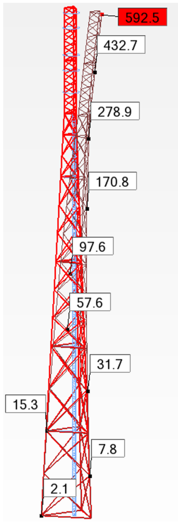
Pav. 17. Maksimalūs lenkimo momentai Mz bokšto stiebo kojose, pagal apkrovų kombinacijų gaubtinę.
