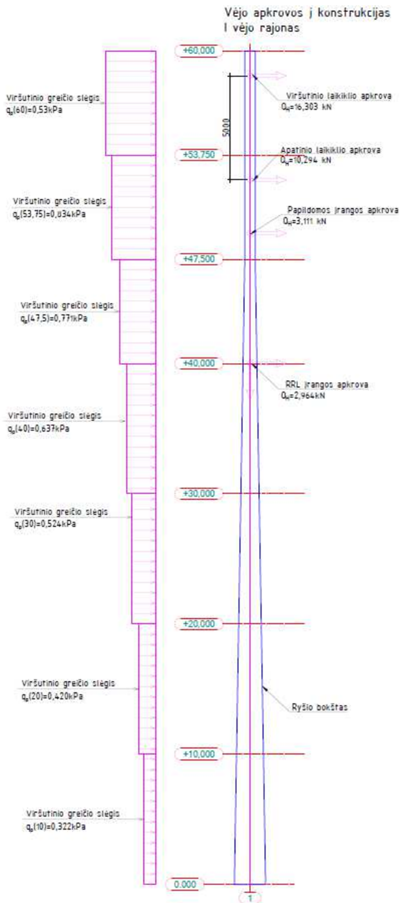
Pav. 5 Bokštą veikiančių apkrovų supaprastinta schema.
