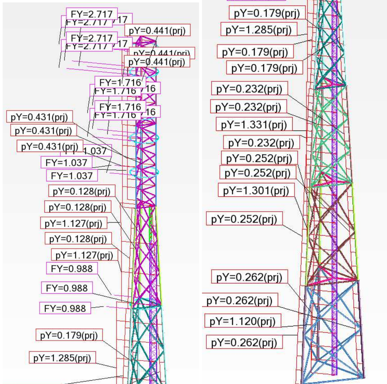
Pav. 10. Vėjo apkrova, 0 laipsnių kryptis. [kN, kN/m] LC4
