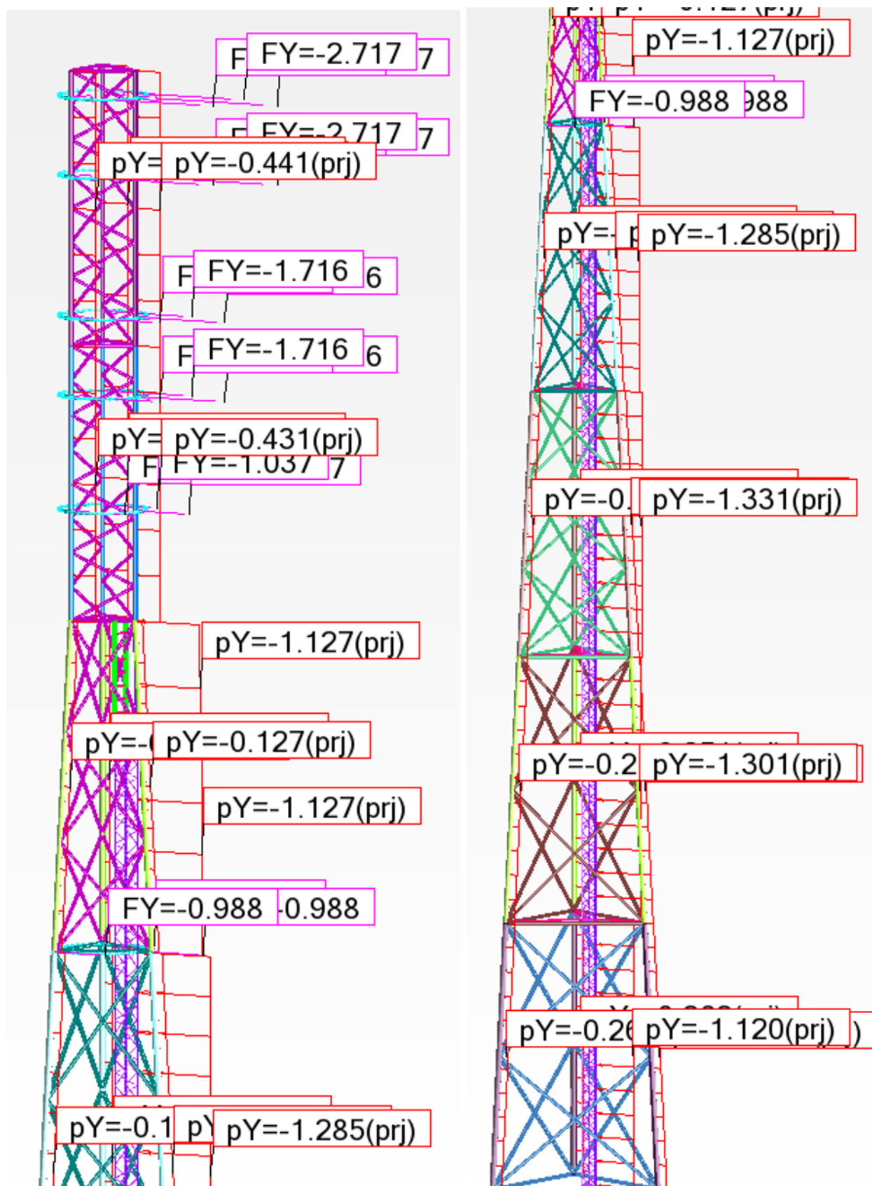
Pav. 12. Vėjo apkrova, 180 laipsnių kryptis. [kN, kN/m] LC6
