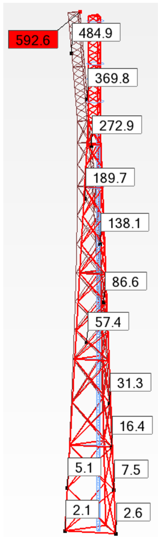
Pav. 19. Maksimalios bokšto deformacijos, pagal charakteristinę CO_S3 apkrovų derinį (vyraujantis vėjas 90 laipsnių kryptis).
