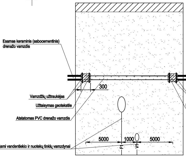
PRINCIPINĖ PAŽISTO DRENAŽO DN50-100 ATSTATYMO DETALĖ
