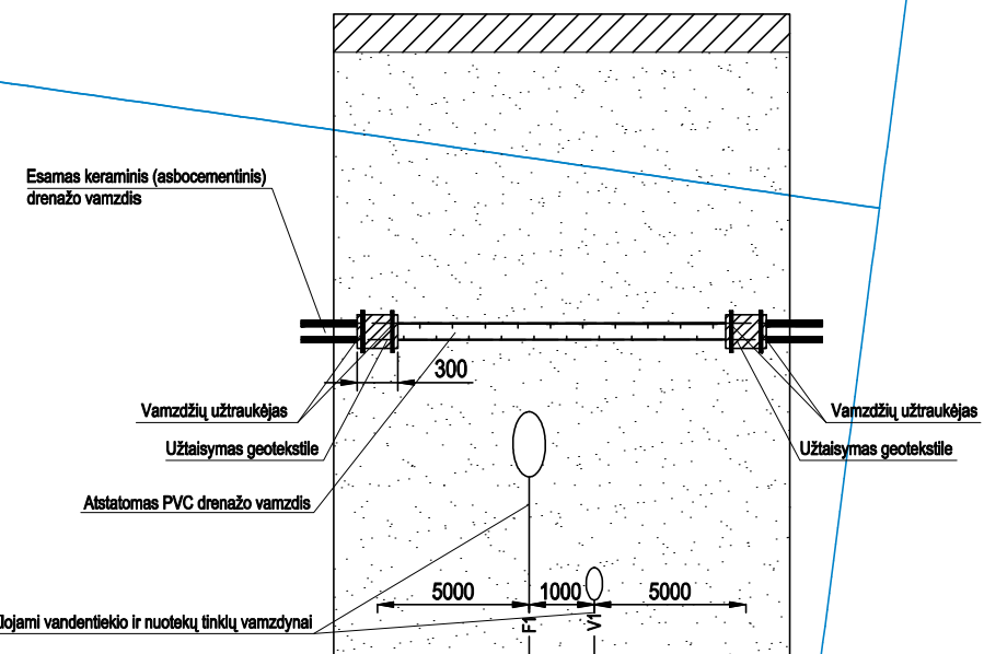
PRINCIPINĖ PĄŽEISTO DRENAŽO DN50-100 ATSTATYMO DETALĖ
