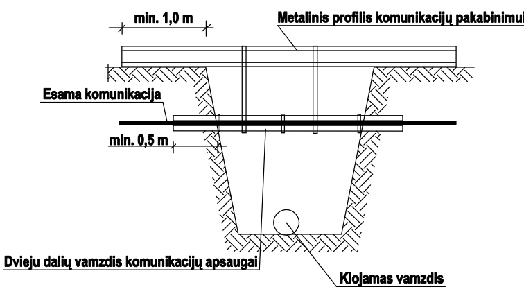
ESAMŲ KOMUNIKACIJŲ PAKABINIMO SCHEMA
