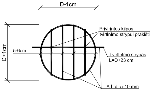
Apsauginių grotelių konstrukcija
