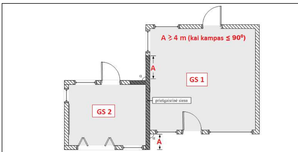
1 pav. Vertikalus ugnies plitimo ribojimo reikalavimai, kur A – priešgaisrinės sienos, atitinkančios REI-M 90 . GS1 – statinys, gaisrinis skyrius Nr. 1 (projektuojamas statinys); GS2 – statinys, gaisrinis skyrius Nr. 2 (priblokuotas esamas statinys).
