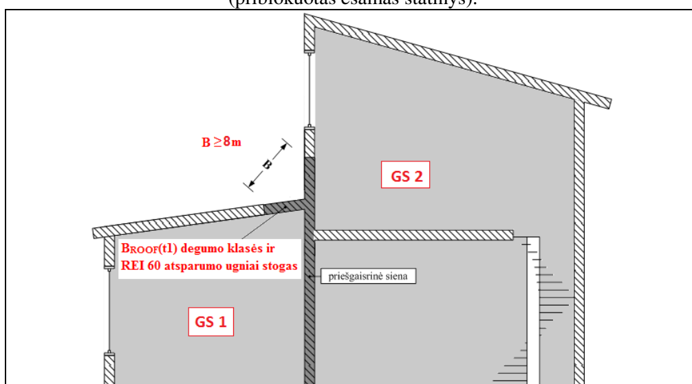
2 pav. Blokuojamų statinių pjūvis, kur B – minimalus stogo, kuris atitinka ne mažesnio kaip REI 60 atsparumo ugniai ir Broof(t1) degumo klasės, matmuo. GS1 – statinys, gaisrinis skyrius Nr. 1 (projektuojamas statinys); GS2 – statinys, gaisrinis skyrius Nr. 2 (priblokuotas esamas statinys).
