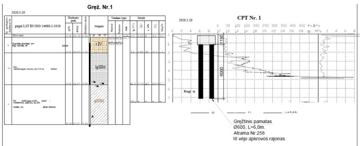
Pav. 1. Konstrukcinė pamatų schema ant geologinio pjūvio
