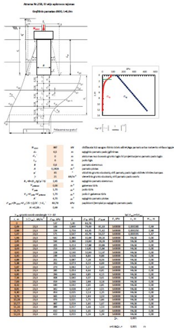
Pav. 8. Poliaus nuosėdžio skaičiavimas
