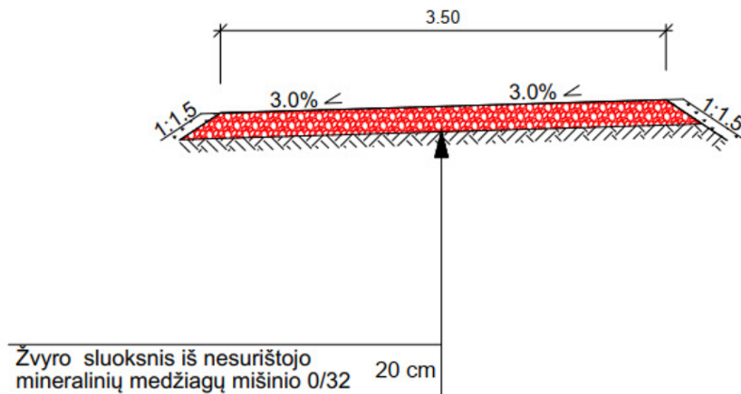
2 pav. Laikino privažiavimo dangos konstrukcija
