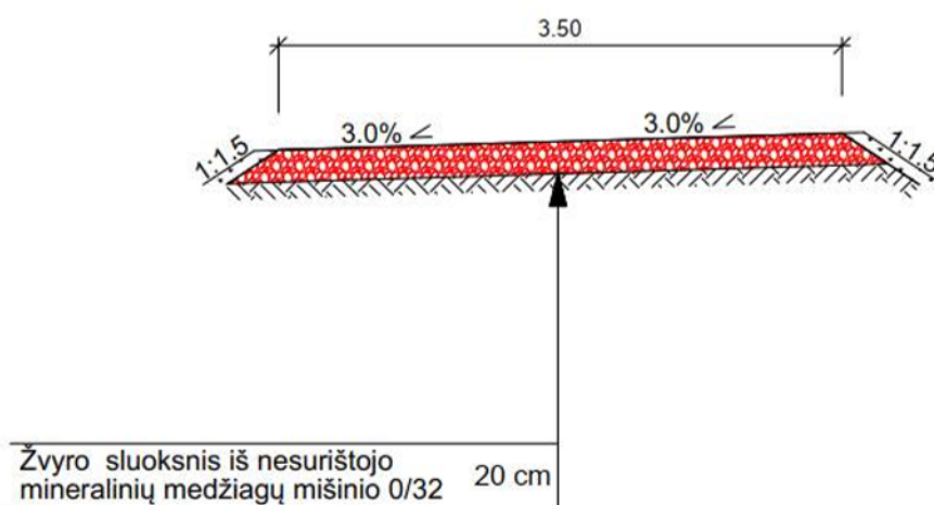
2 pav. Laikino privažiavimo dangos konstrukcija
