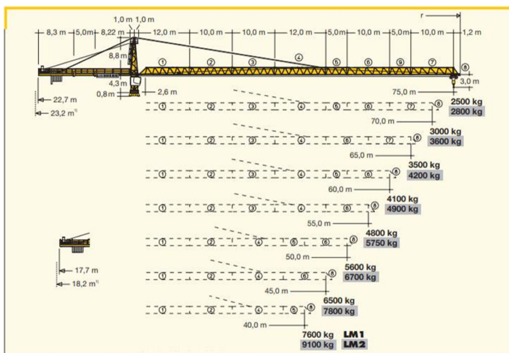
Liebherr 280 EC-H kėlimo galios schema
