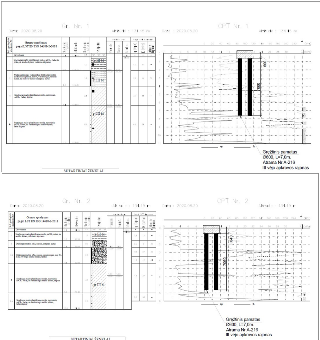
Pav. 1. Konstrukcinė pamatų schema ant geologinio pjūvio
