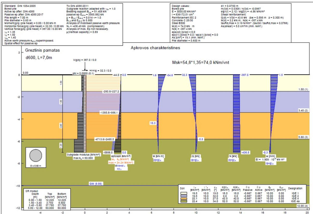
Pav. 5. Poliaus laikomosios galios tikrinimas nuo skersinės jėgos sudaromo momento
