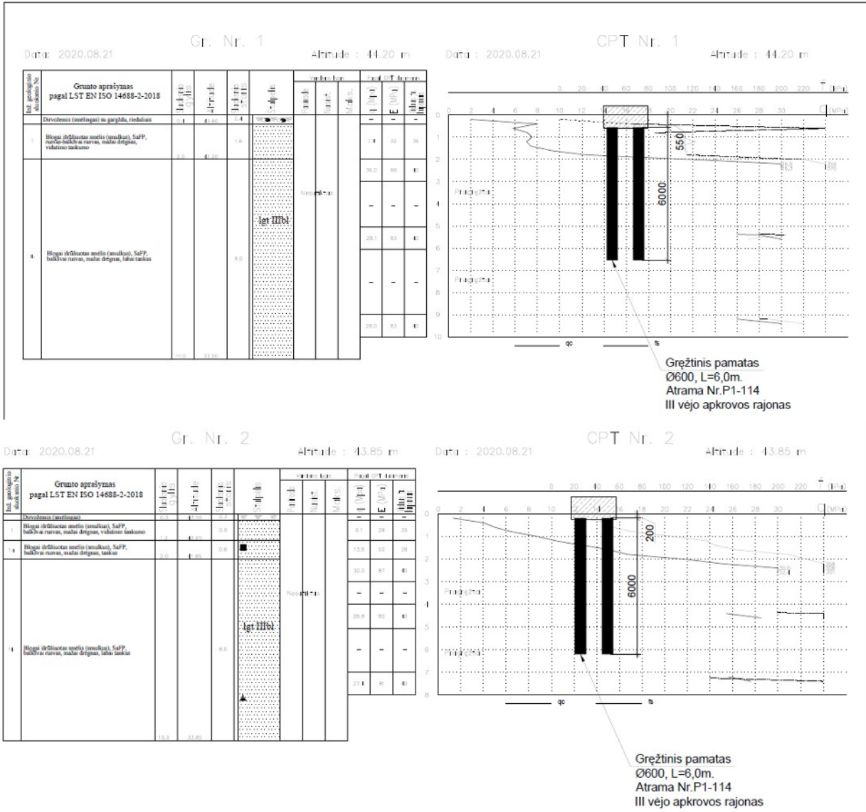
Pav. 1. Konstrukcinė pamatų schema ant geologinio pjūvio
