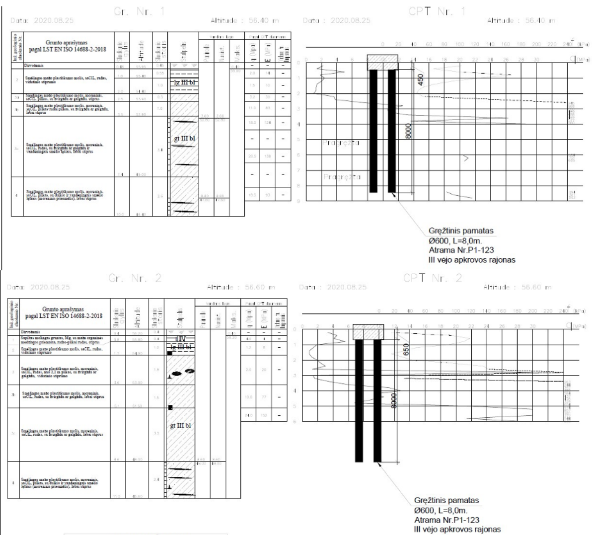
Pav. 1. Konstrukcinė pamatų schema ant geologinio pjūvio
