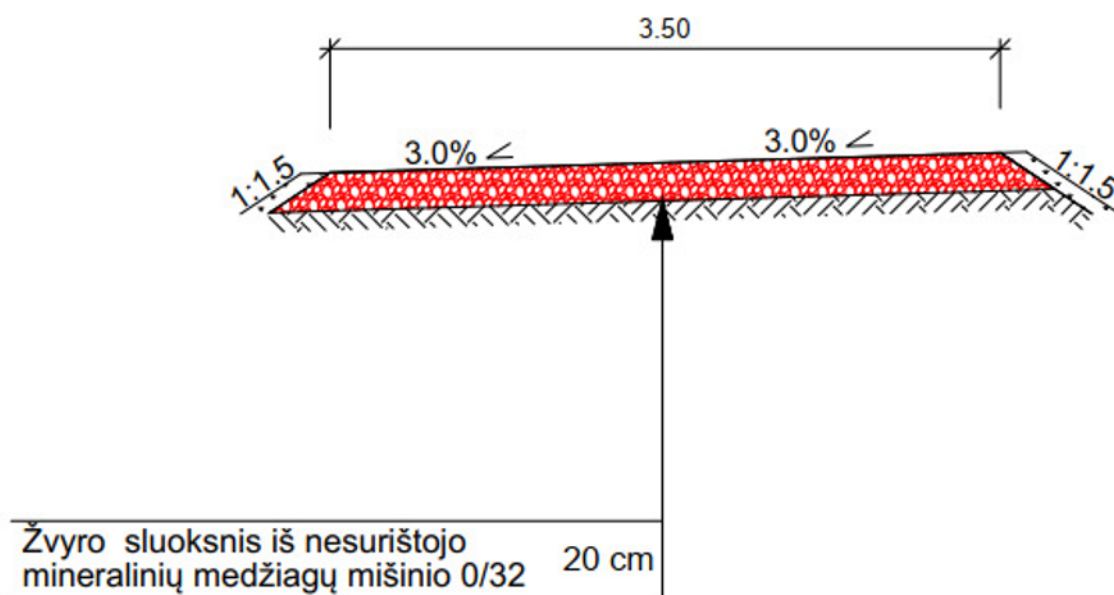
2 pav. Laikino privažiavimo dangos konstrukcija
