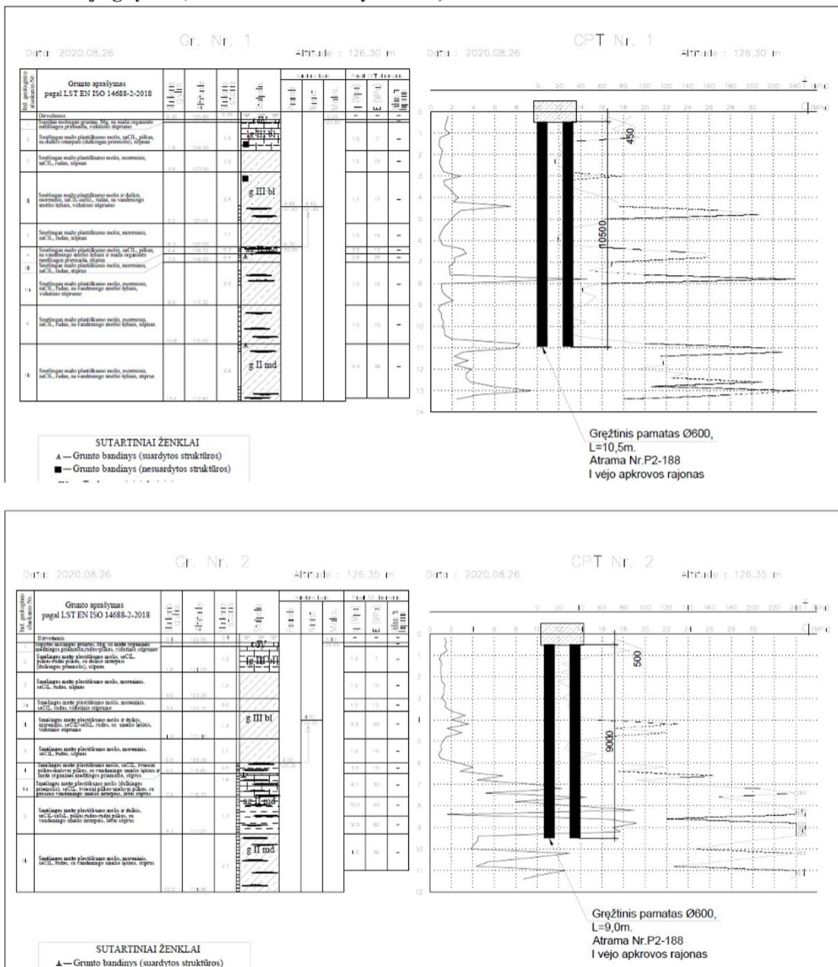
Pav. 1. Konstrukcinė pamatų schema ant geologinio pjūvio
