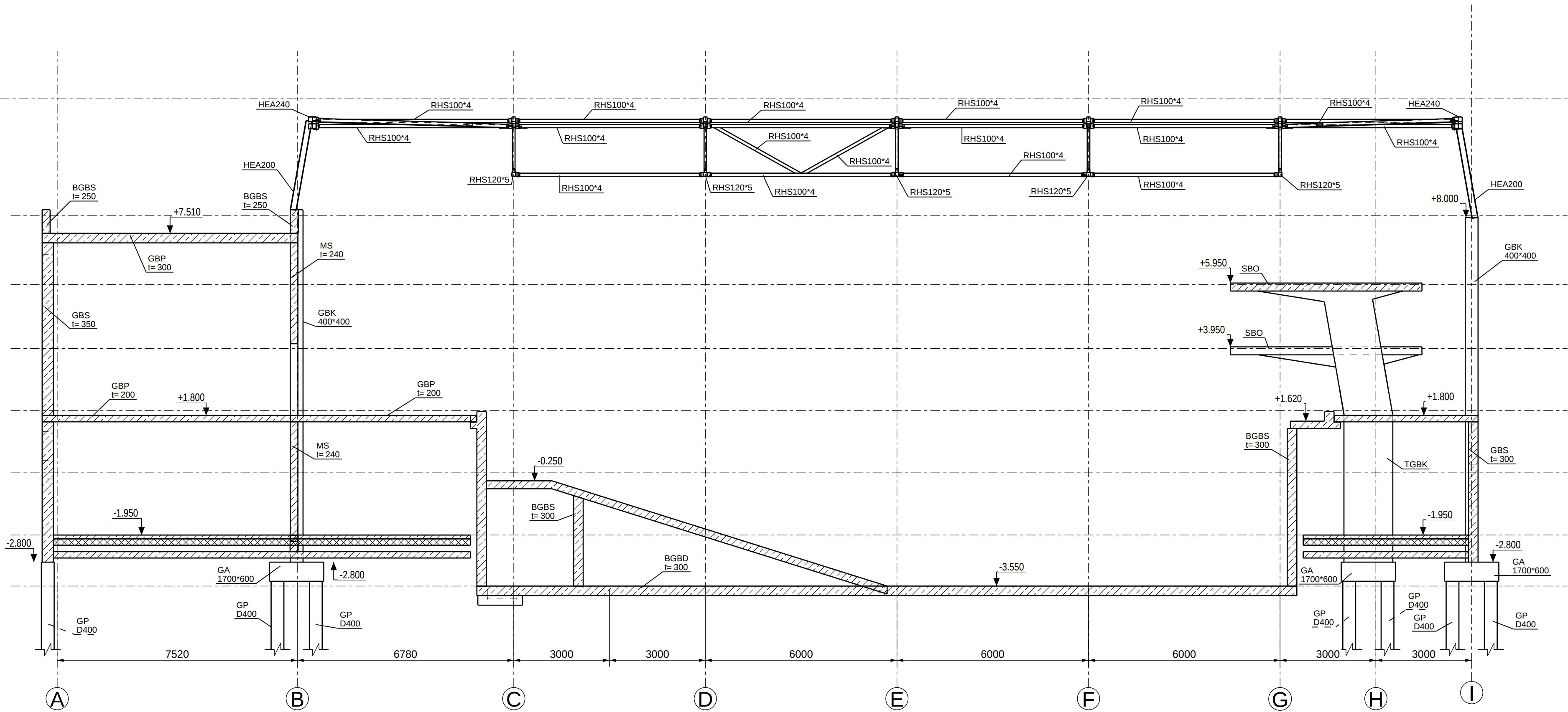
PŪVIS 3-3 AŠYJE 1:100
