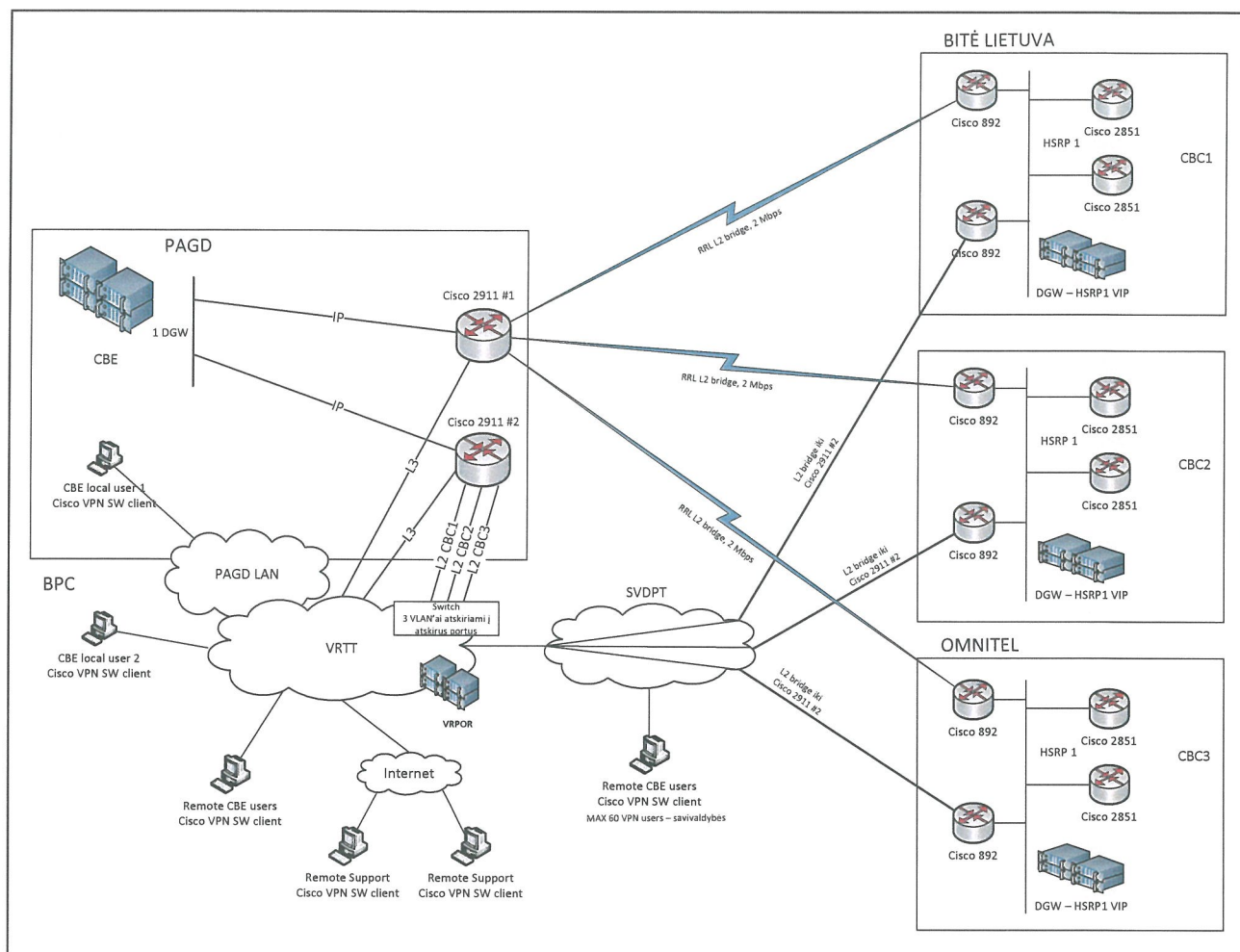
4 pav. GPIS posistemių jungiamojo tinklo architektūra
