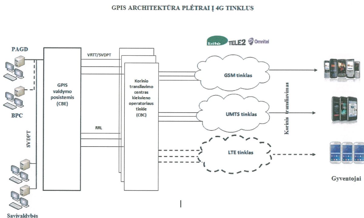
1 pav. GPIS architektūra
