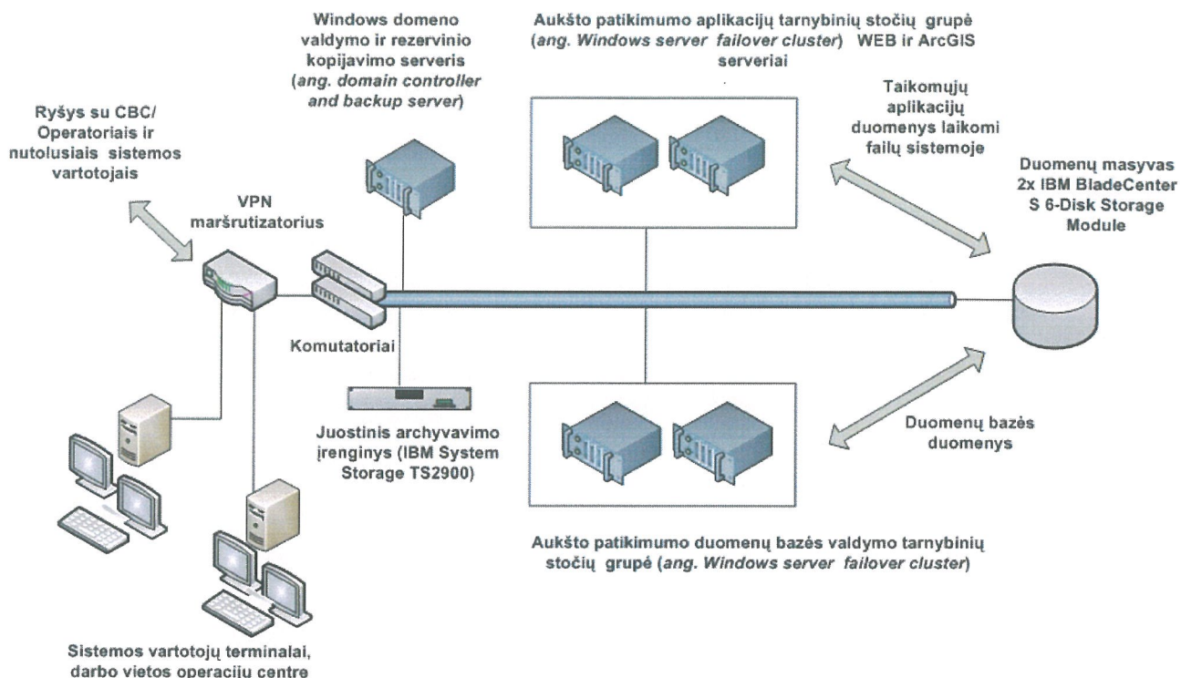
2 pav. CBE posistemo architektūra
