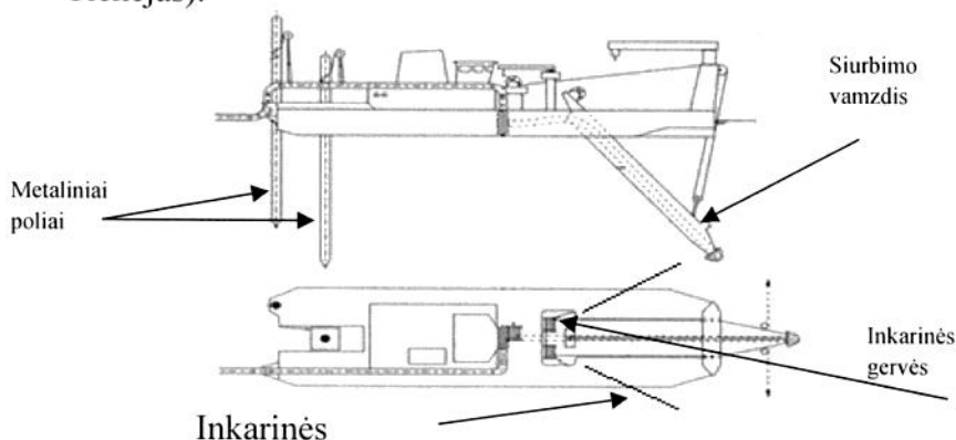
1 pav. Žemsiurbės principinė schema.
