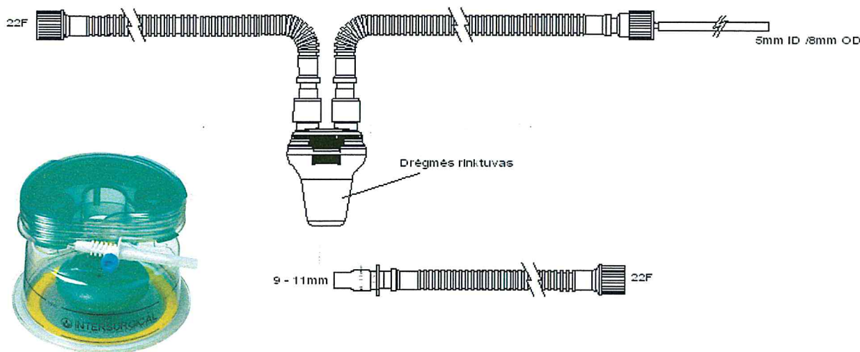
Automatiškai prisipildantis deguonies drėkinimo indas (Gaminio kodas 2310000)
