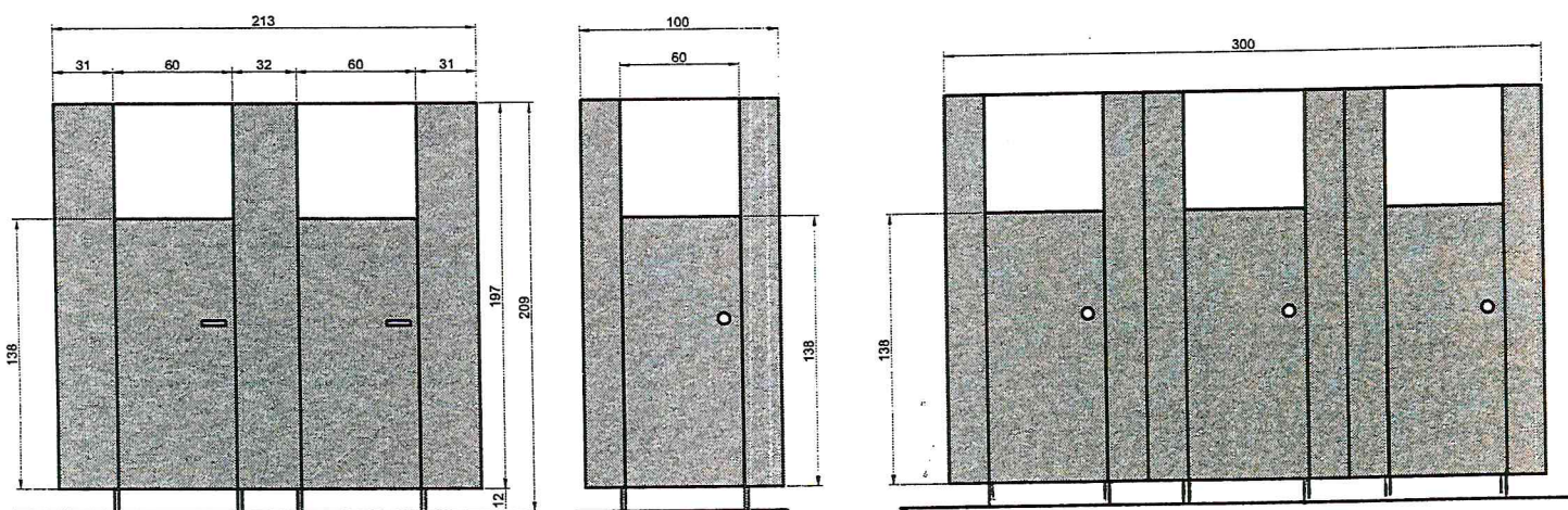
1 pav. Pertvarų montavimo schema
