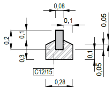
VEJOS BORDIŪRO SU PAMATU DETALĖ 100X8X20
