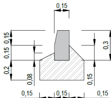
KELIO BORDIŪRO SU PAMATU 100x15x30
