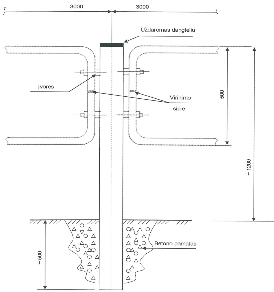
PĖSČIŲJŲ ATITVARO STULPELIO IR SEKCIJOS BRĖŽINYS Nr. 1.
