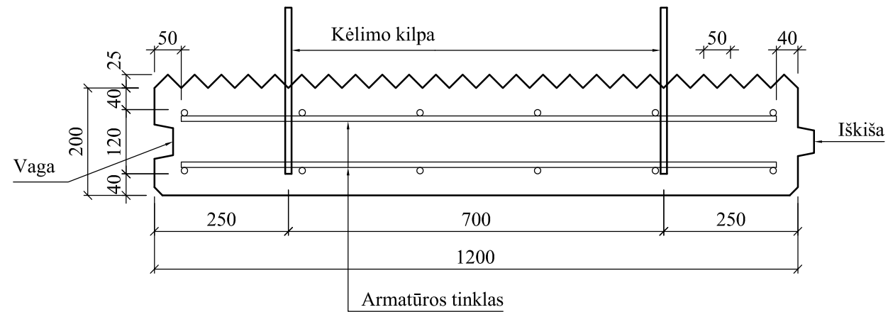
4 - 4 M 1:10
