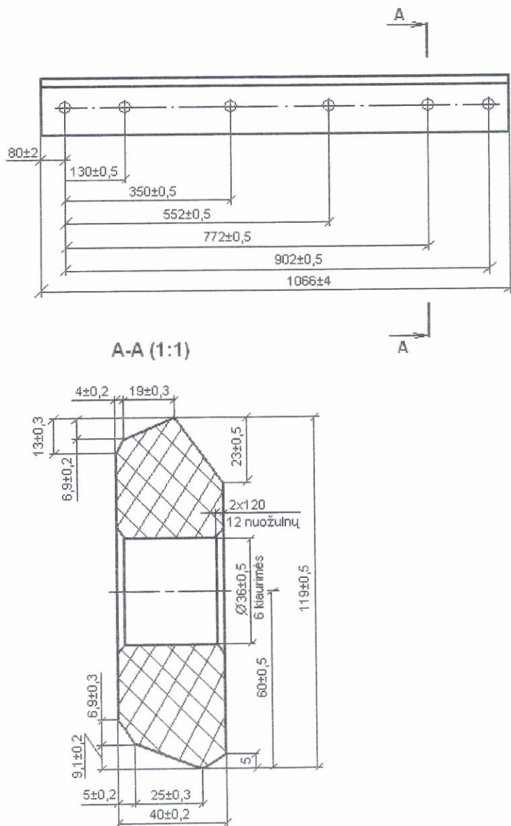
3 brėžinys. Plastikinė tvarslė UIC60 (60E1) (6 skylių)
