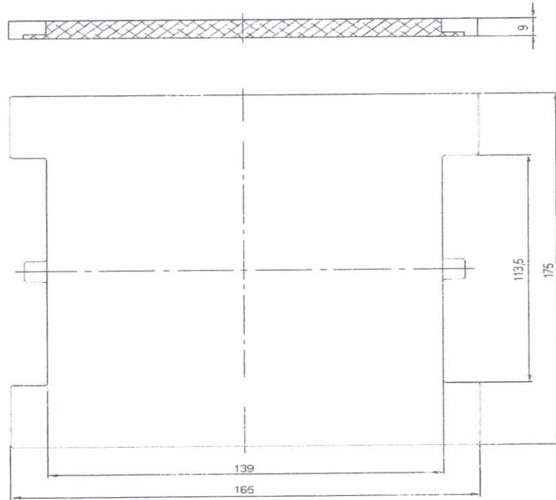
4 brėžinys. Tarpiklis po bėgiu R65 SKL14
