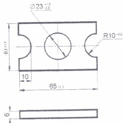
3 brėžinys. Plokščia poveržlė
