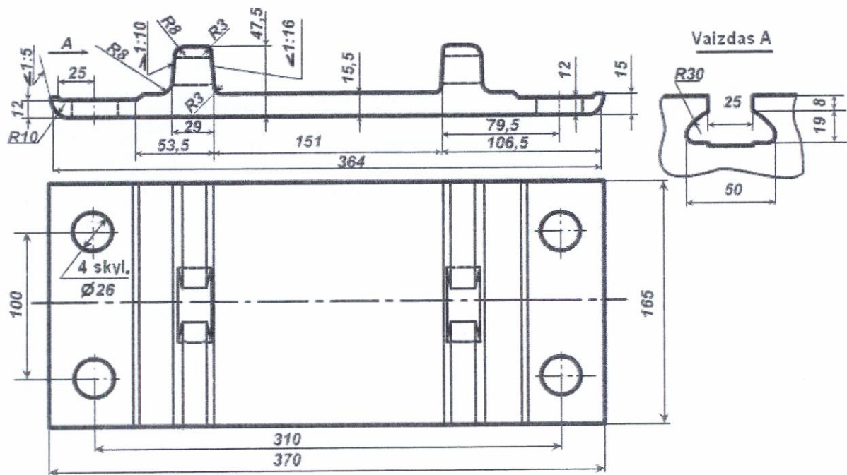
5 brėžinys. Mišrių sąvaržų padėklas SK R65 (iešminis)
