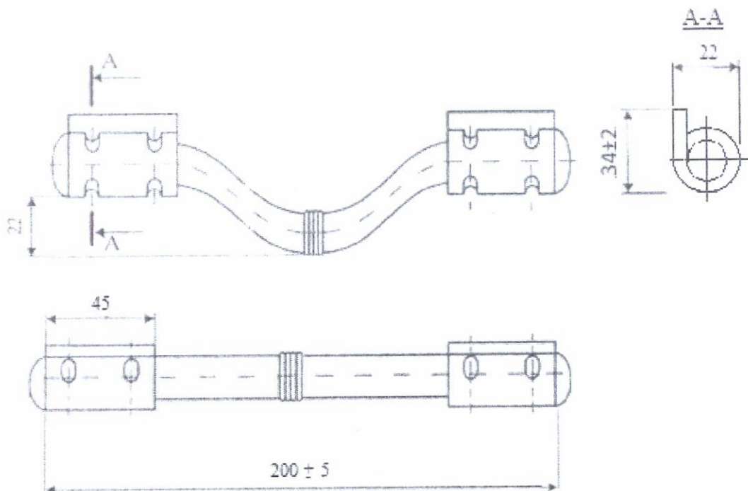
10 brėžinys. Varinė sandūrinė privirinama jungė
