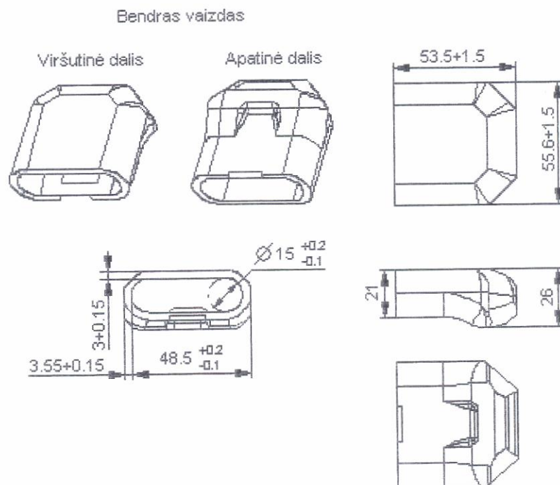
13 brėžinys. Antgalio izoliatorius (f-clip)
