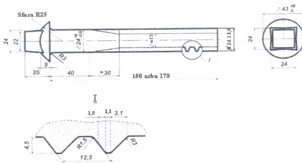
6 brėžinys. Medsraigtis 1.24x150 ir 1.24x170
