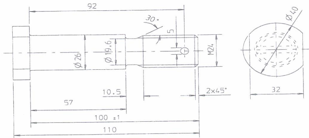
7 brėžinys. Velenėlis
