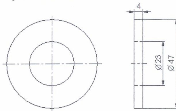
18 brėžinys. Poveržlė Uls 6
