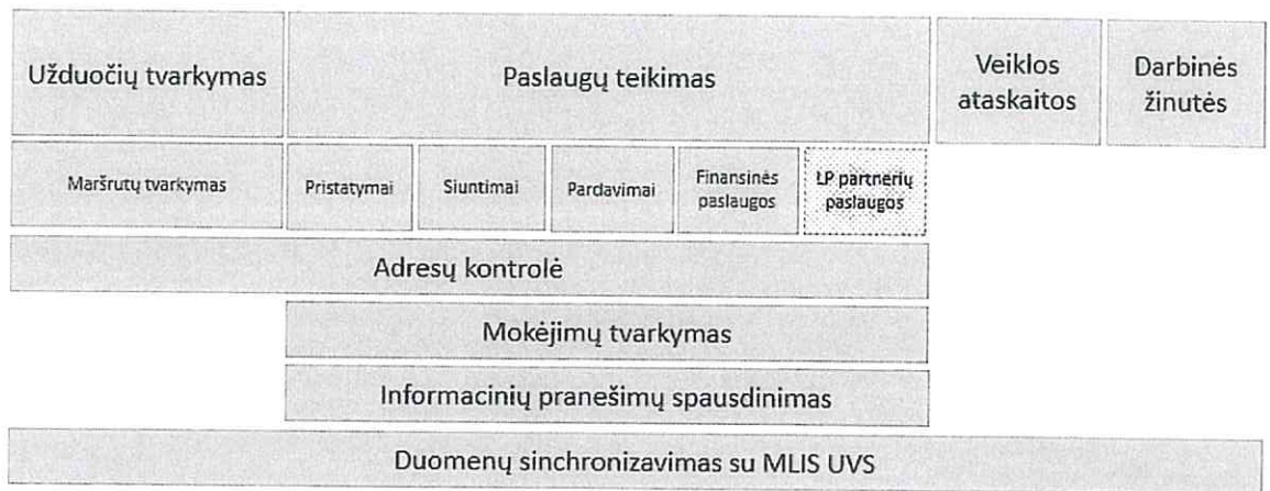
Figūra. Pvz.: mobilaus laiškinko sistemos Mobilios programėlės posistemės funkciniai moduliai
