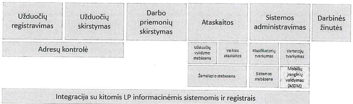
Figūra. Pvz.: mobilaus laiškinko sistemos Užduočių valdymo posistemės funkciniai moduliai
