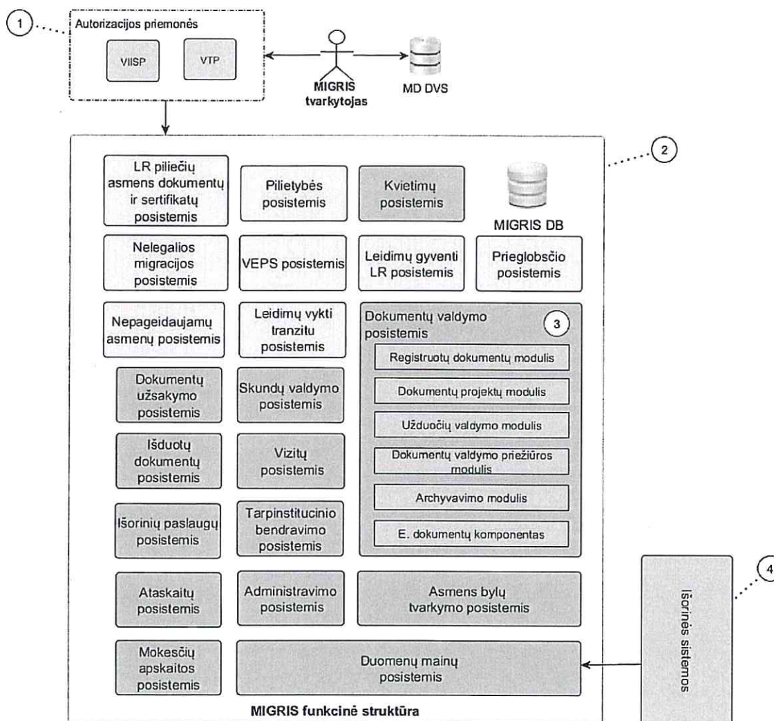
1 paveikslas. Konceptinė MIGRIS funkcinės architektūros schema
