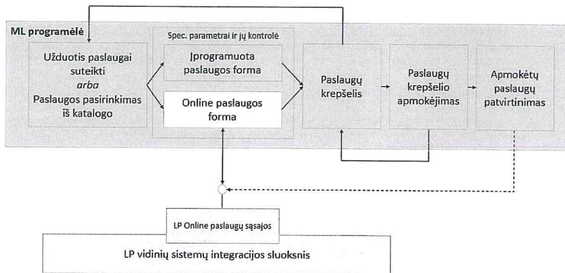
Figūra. Pvz.: mobilaus laiškinių programėlės sąveikos su online įskiepiais bendra architektūra
