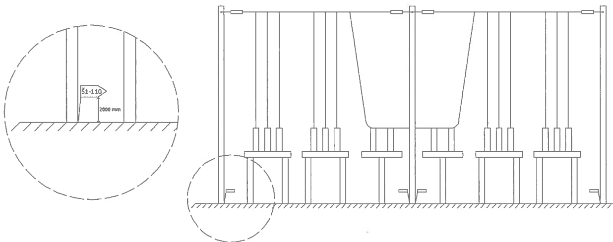
1 pav. ŠyŲ sekcijŲ žymėjimas esant lanksčioms šyŲoms
