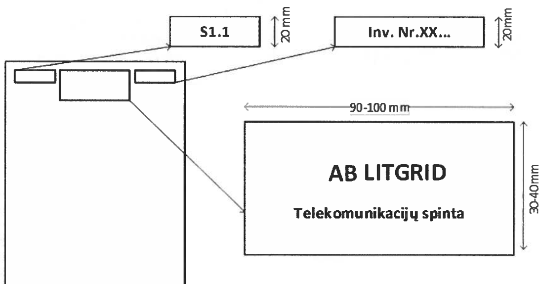
1 pav. Telekomunikacijų spintos žymėjimo etiketės pavyzdys
