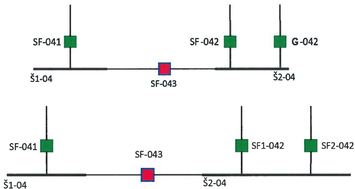
1 pav. Dviejų savųjų reikmių 0,4 kV šynų sekcijų komutacinių aparatų operatyvinių pavadinimų pavyzdžiai
