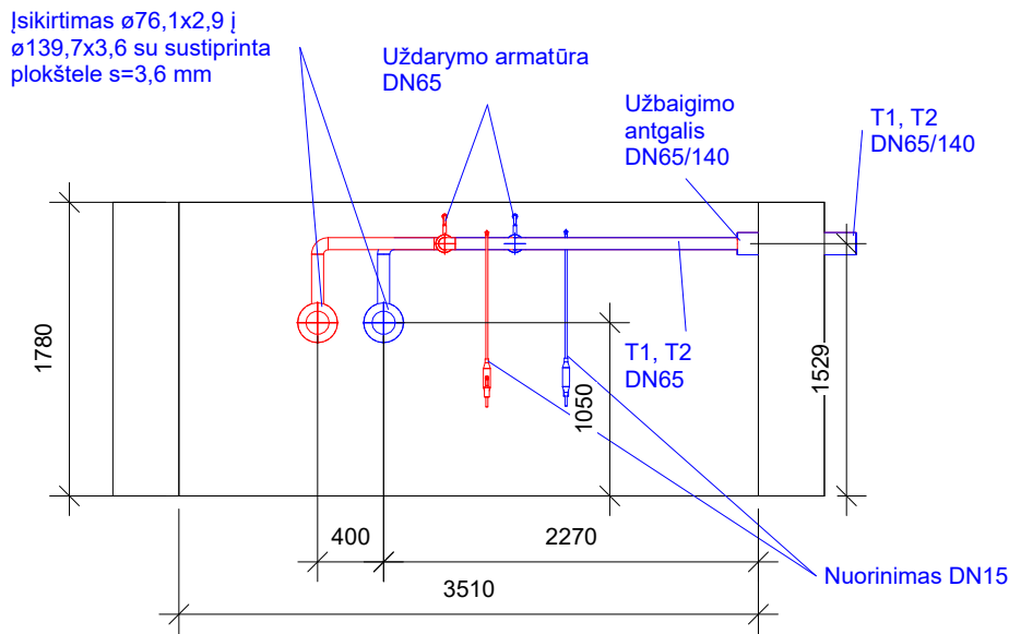
Pjūvis 2-2 M 1:50
