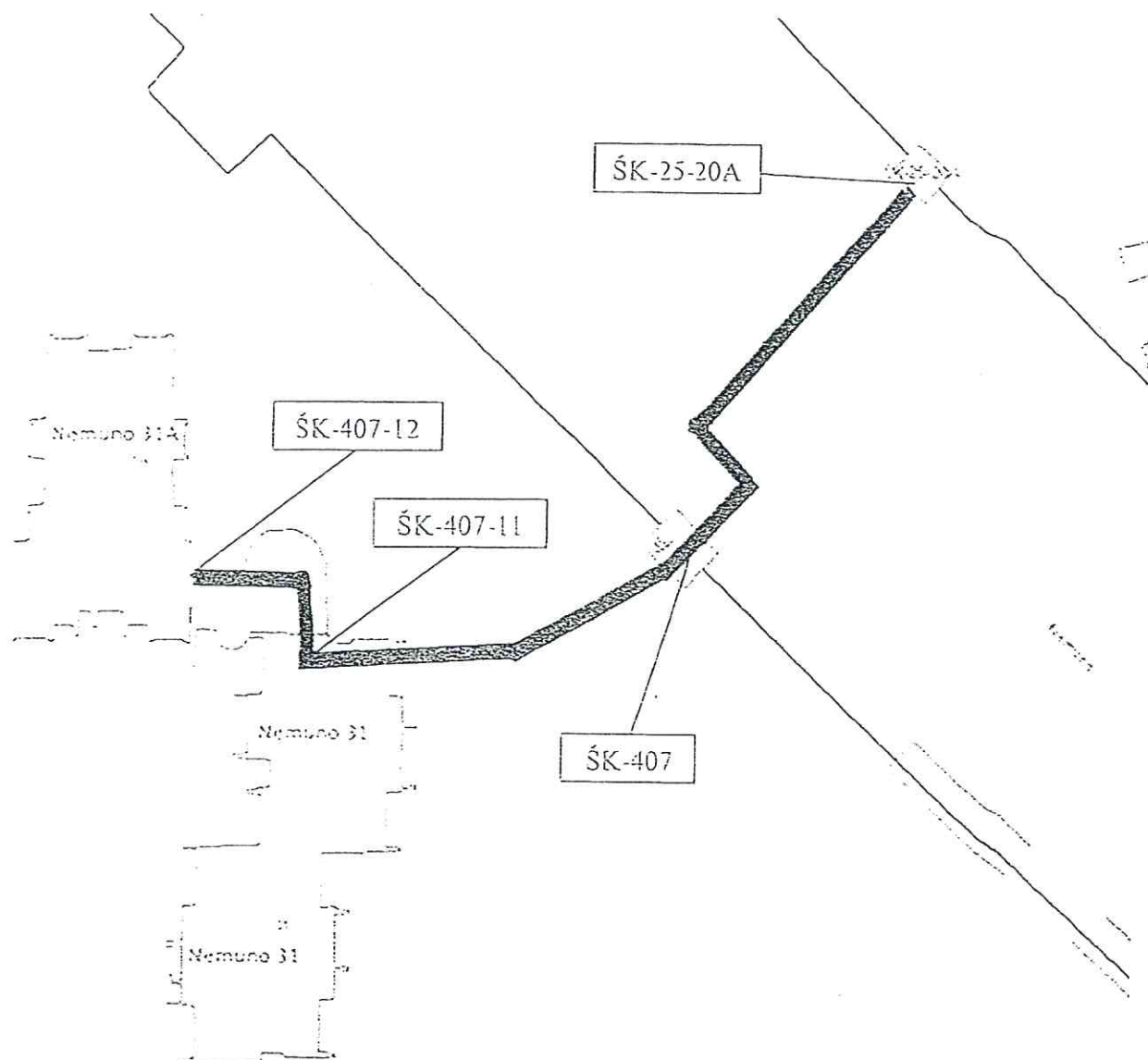
Šilumos tinklų nuo ŠK-25-20A iki Nemuno g. 31a situacijos schema
