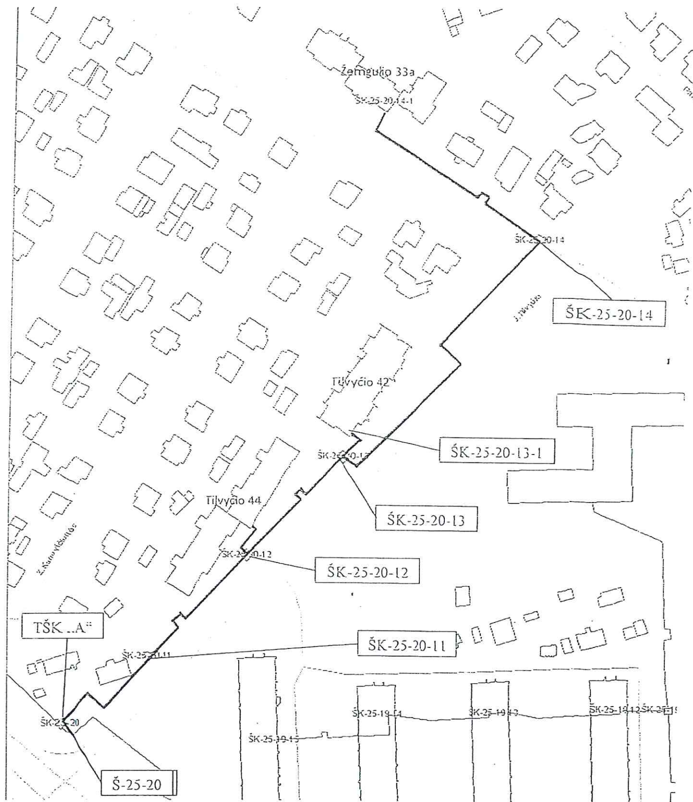
Šilumos tinklų nuo TŠK „A“ prie ŠK-25-20 iki J. Žemgūlio g. 33a su atšakomis situacijos schema
