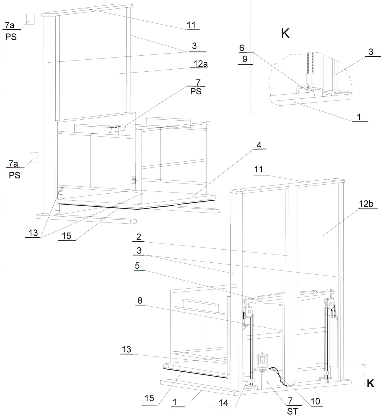
brėž. 1 Įrenginys / hidraulinis keltuvas/, skirtas neįgalių asmenų pervežimui vertikalus DHP tipo / / įvažiavimas ir išvažiavimas 90° kampu /
