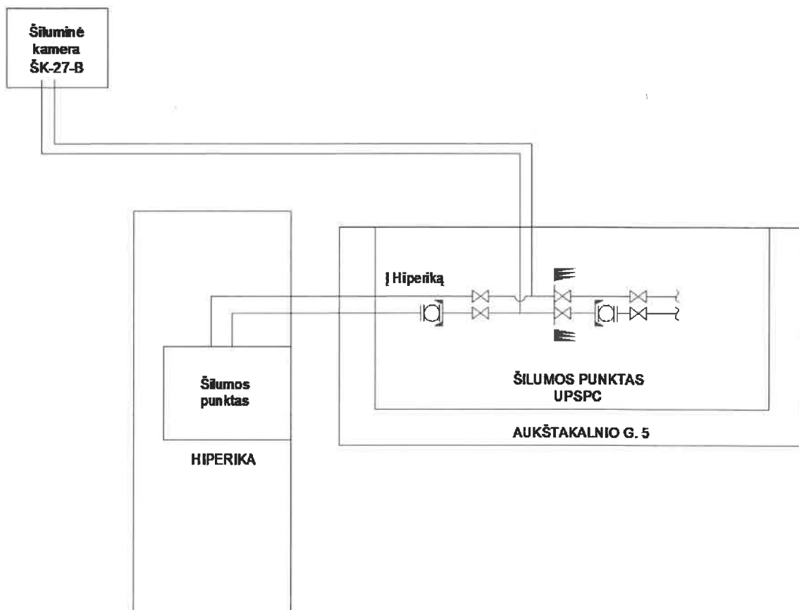
Šilumos įrenginių schema:
