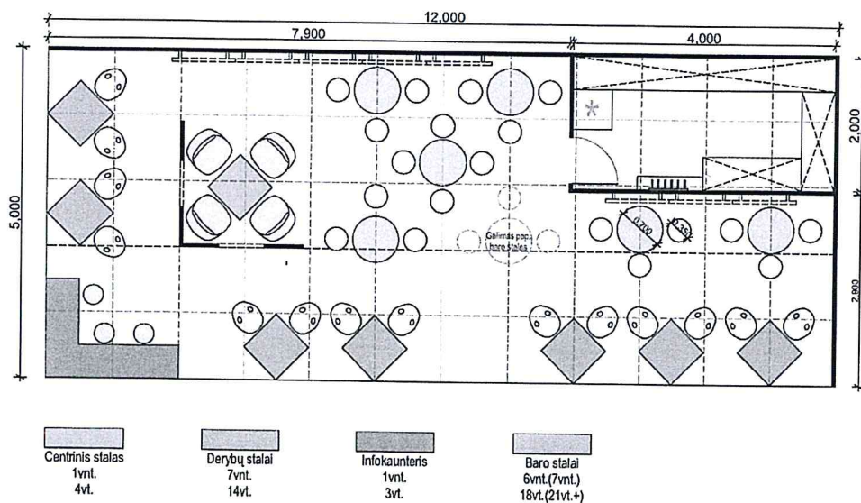
STENDO PLANAS M 1:50
