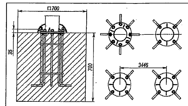
Ankerių tvirtinimo prie bazono schema
