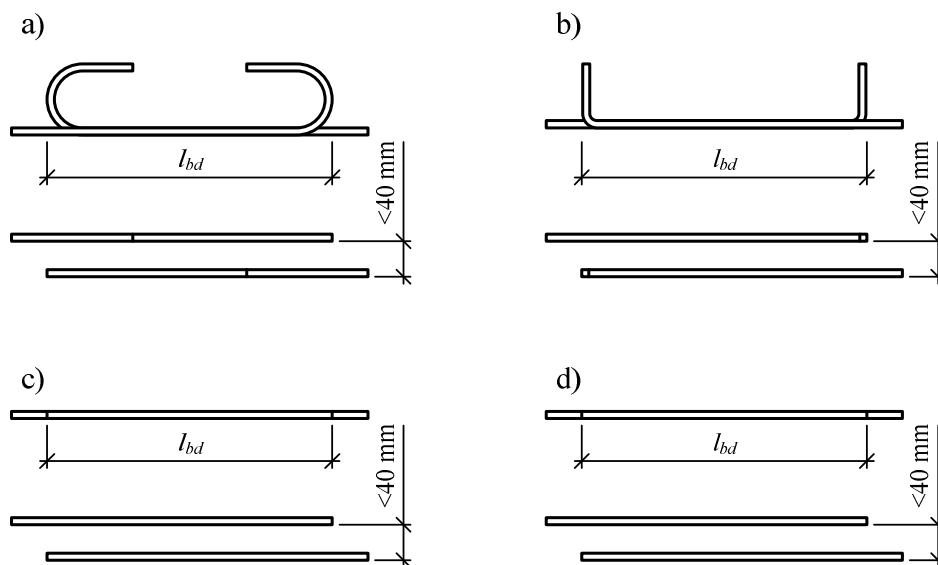
1 paveikslas. Strypų sujungimas užlaida be suvirinimo (a, c – lygios armatūros; b, d – rumbuotosios)
