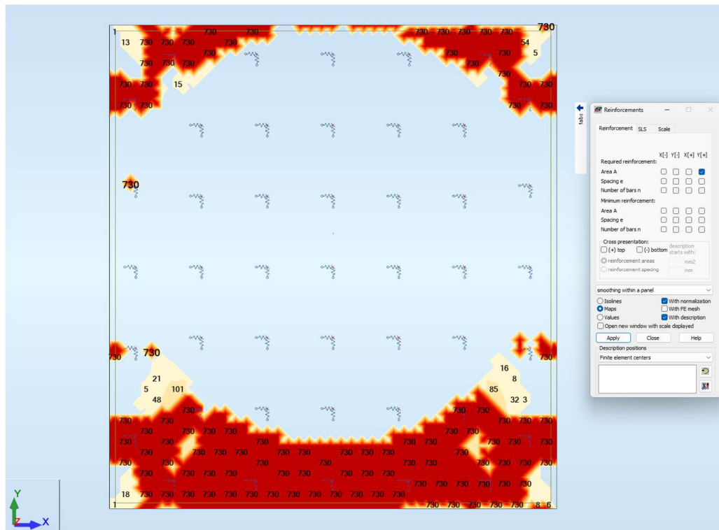
7 pav. Viršutinio tinklo reikiamas armatūros kiekis Y-Y kryptimi (mm²/m).
