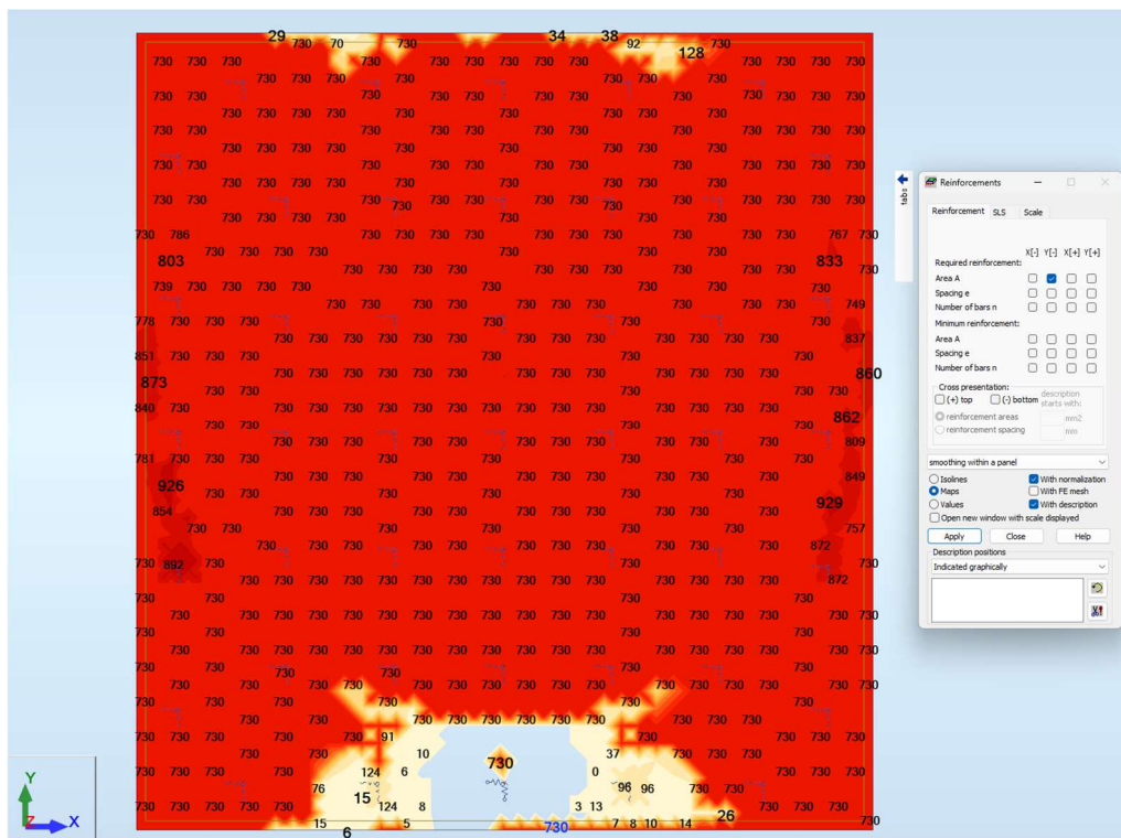
5 pav. Apatinio tinklo reikiamas armatūros kiekis Y-Y kryptimi (mm²/m).
