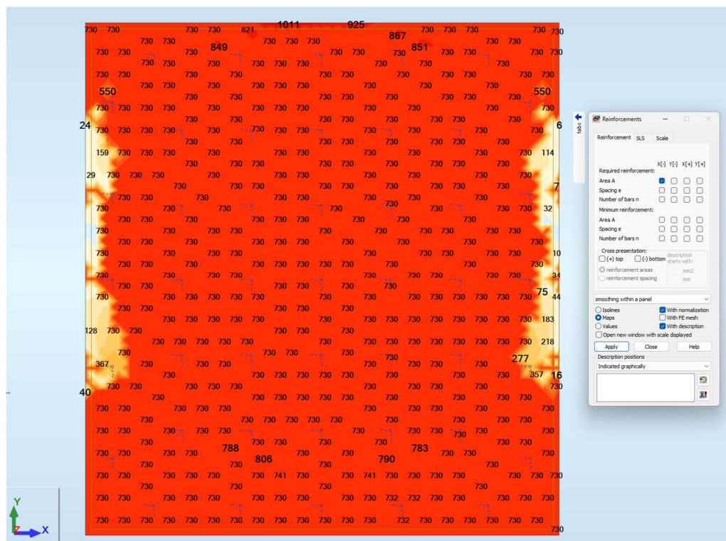
4 pav. Apatinio tinklo reikiamas armatūros kiekis X-X kryptimi (mm²/m).
