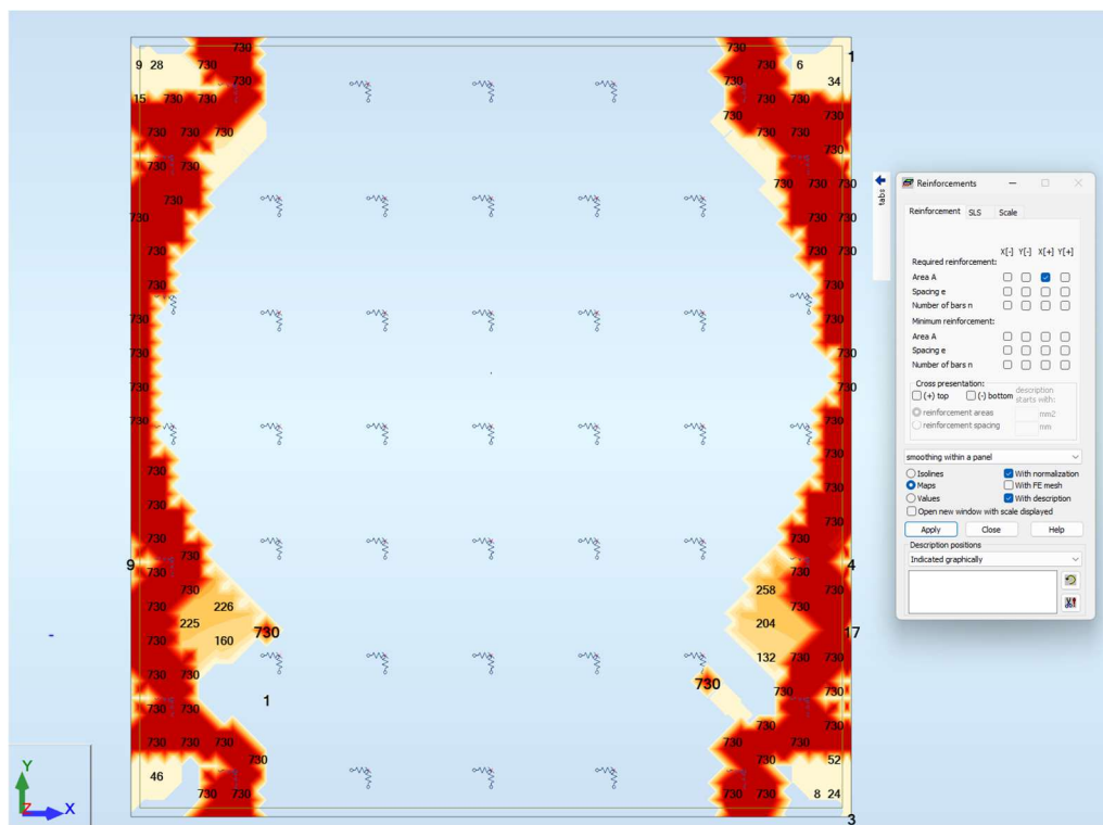
6 pav. Viršutinio tinklo reikiamas armatūros kiekis X-X kryptimi (mm²/m).
