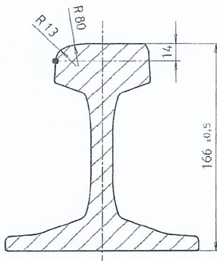
2 paveikslas. Reprofiluoto bėgio skerspjūvis
