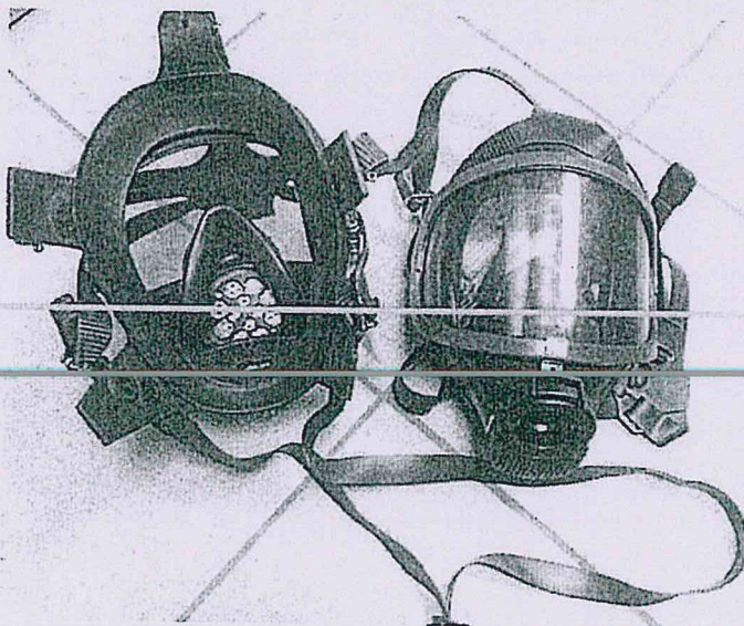
Suspausto oro kvėpavimo kaukės pavyzdinis modelis
