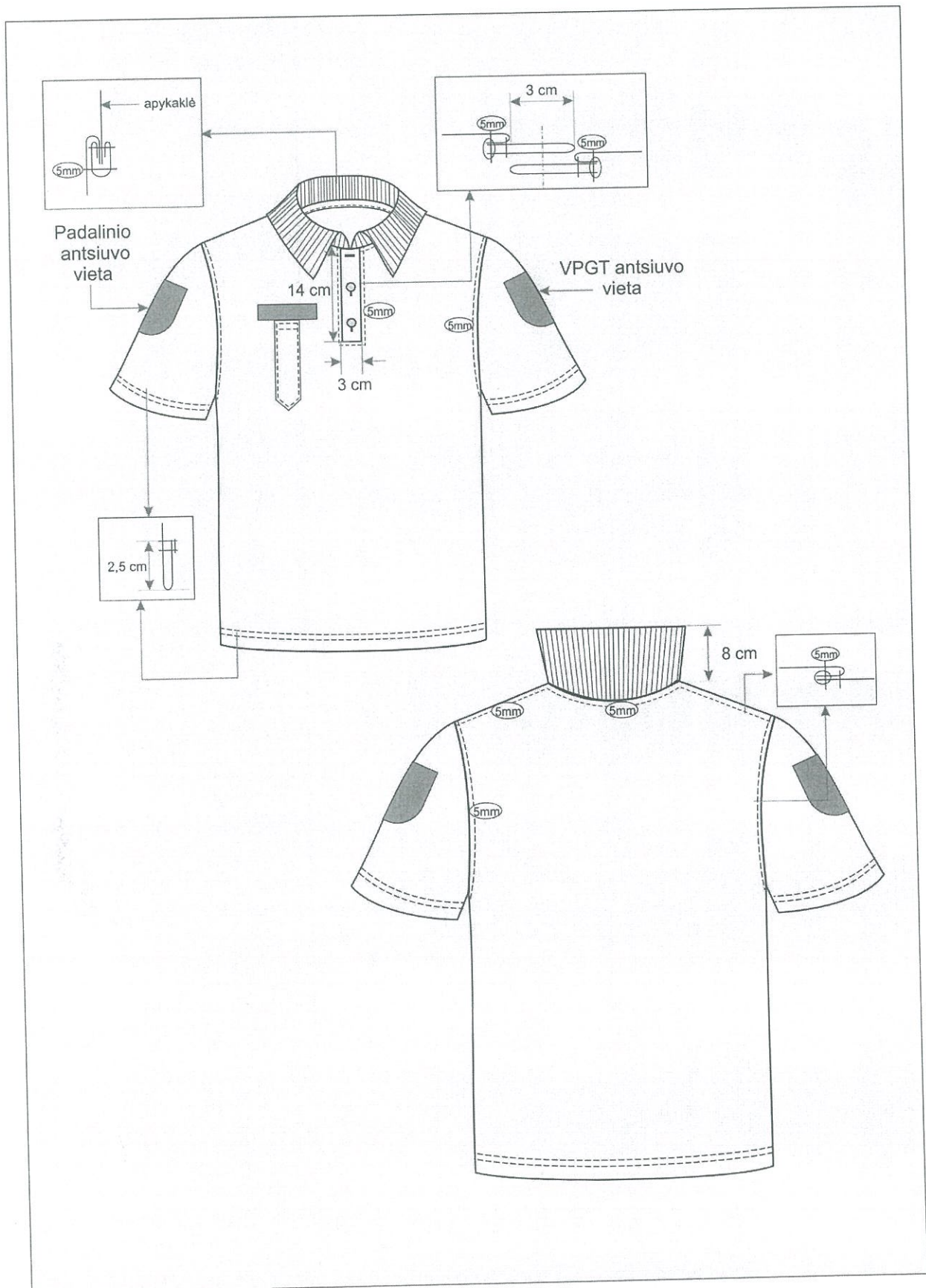
2 pav. Vasarinių marškinėlių techninis brėžinys
