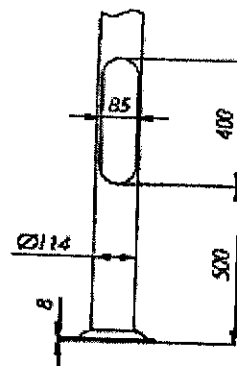
Pav. Nr.2 Atramos durelių pavyzdys
