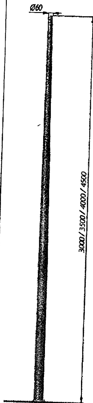
Pav. Nr.1 Atramos pavyzdys
