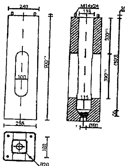
Pav. Nr.4 Atramos pamato pavyzdys
