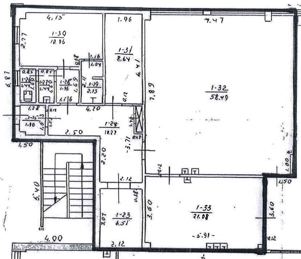
1 pav. Patalpų eksplikacija
