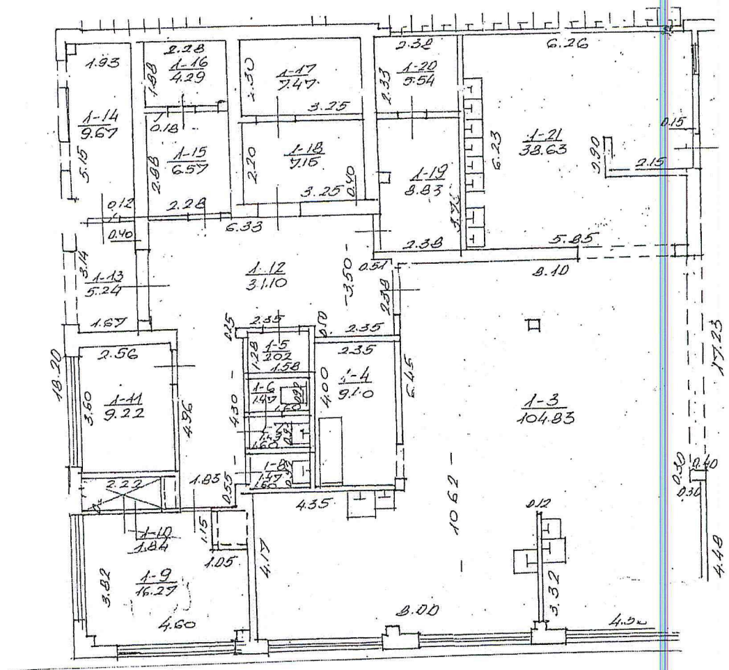
1 pav. Patalpų eksplikacija
