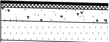
ATSTATOMOS DVISLUOKSNĖS ASFALTO DANGOS (GRUNTO KLASĖ PAGAL JAUTRUMĄ ŠALČIUI - F3) PJŪVIS DK 1
