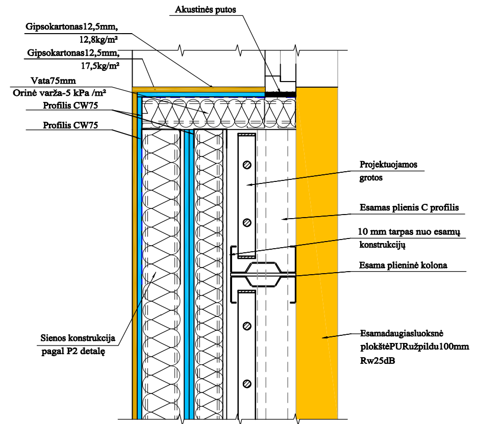
Esamos lauko sienos papildoma garso izoliacija pagal detalę P2 Angokraščio įrengimo mazgas M1:10
