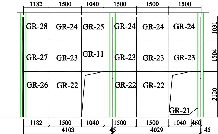
Grotų išdėstymas (5-5) M1:100
