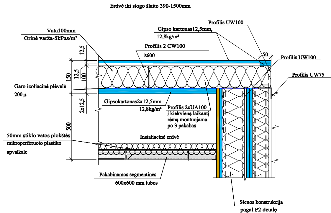
Detalė L1 vertikalus pjūvis Akustinių lubų sujungimo su išorės sienomis mazgas ir papildoma pakabinamų lubų garso izoliacija M1:10
