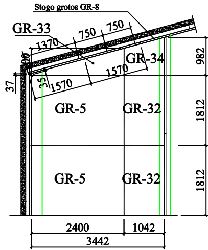
Grotų išdėstymas (3-3) M1:100
