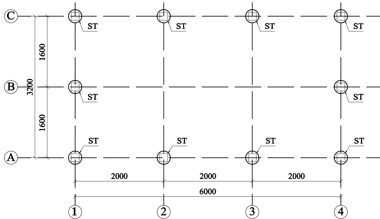
STATRAMSČIŲ PLANAS M1:50
