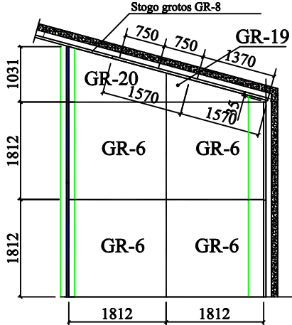
Grotų išdėstymas (4-4) M1:100
