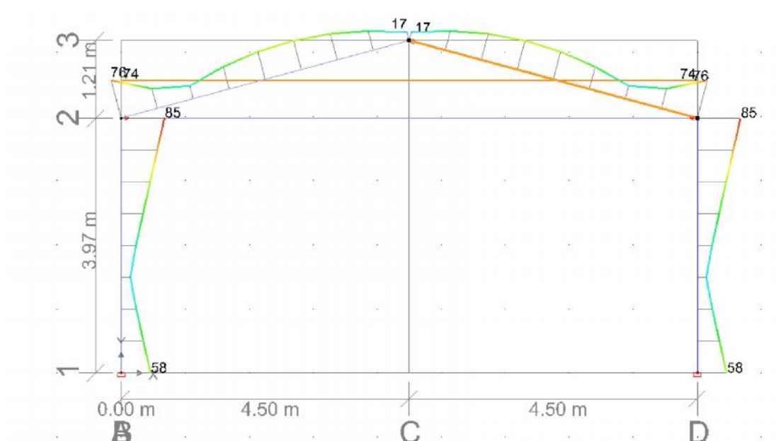
Pav. 3 Bendras išnaudojimas nuo pavojingiausio derinio ULS, 74 proc.
