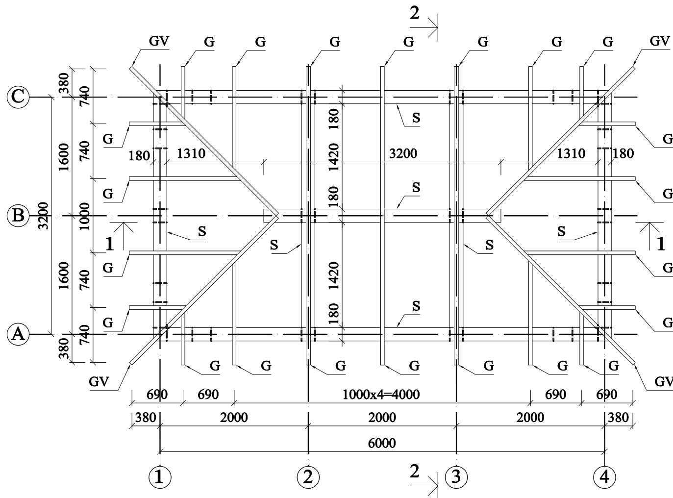
DENGINIO PLANAS M1:50
