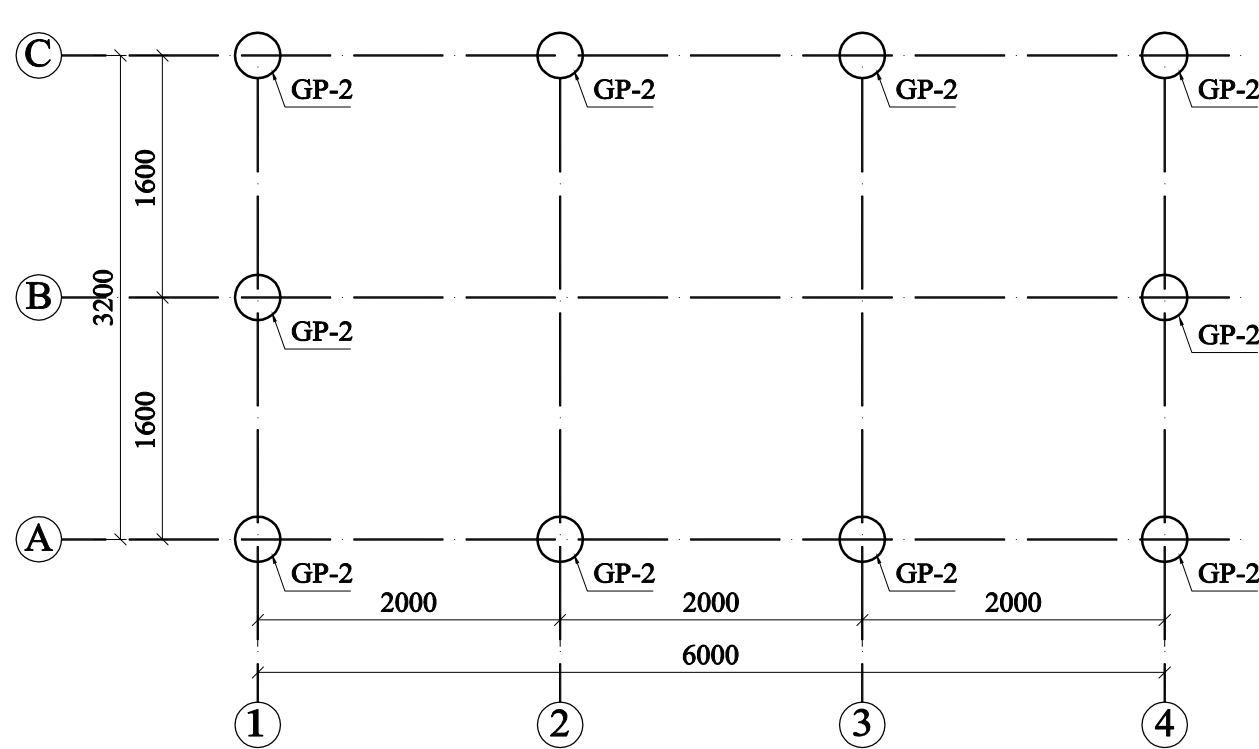
POLIŲ PLANAS M1:50
