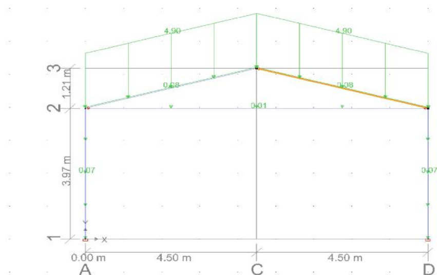
Pav. 2 bendros apkrovos ULS nuo pavojingiausio derinio
