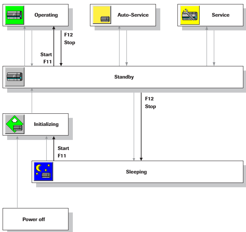
pav. 0-26 Sistemas būsenos (parodytos ne visos būsenos)
