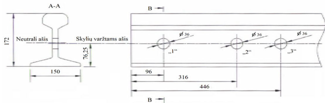
1 priedas. UIC60 (60E1) tipo bėgyje skylių gręžimo nužymėjimo schema
