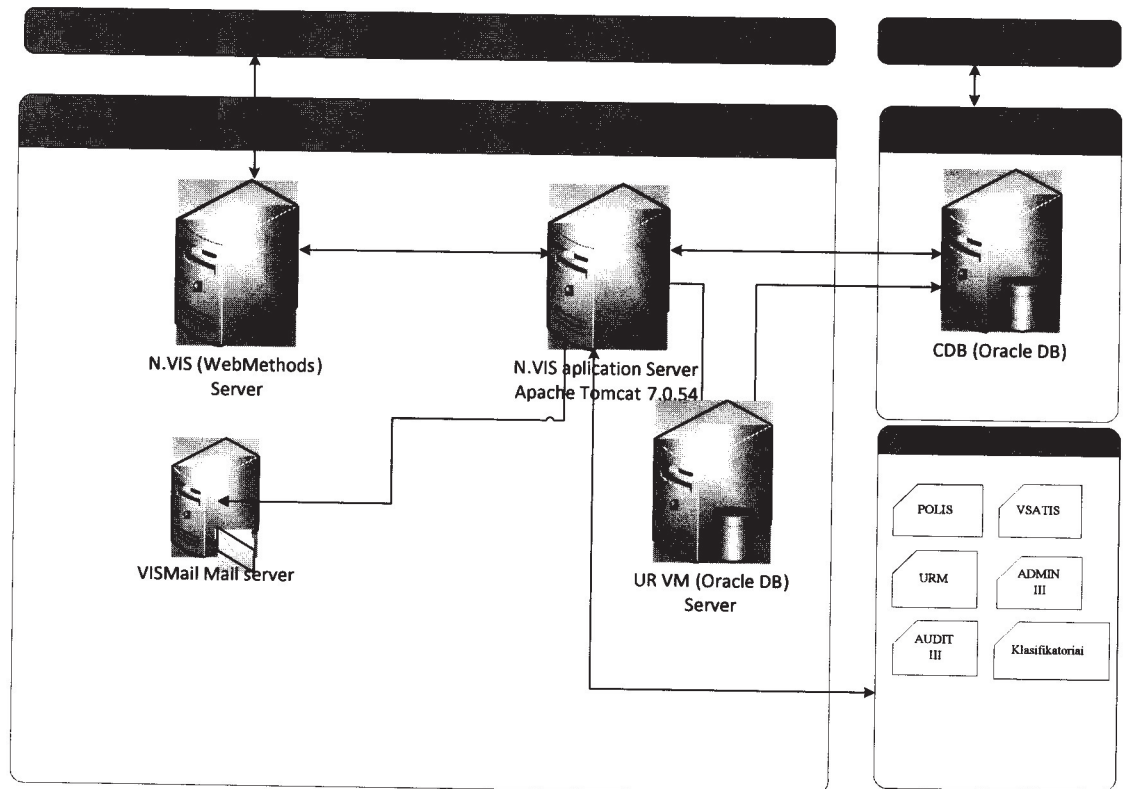
1 pav. N.VIS techninės infrastruktūros schema
