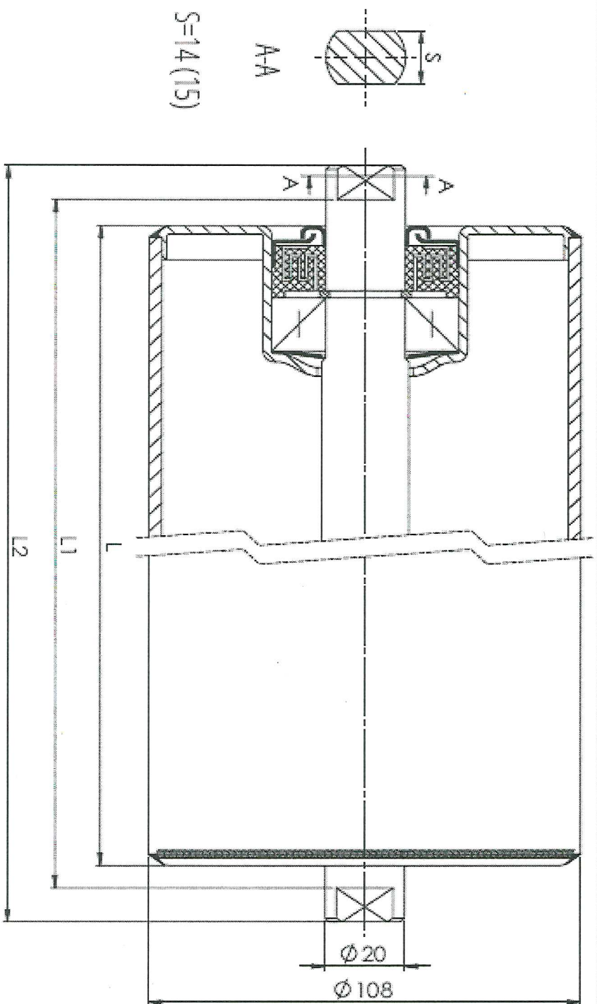
Nešantieji ritinėliai - brėžinys
