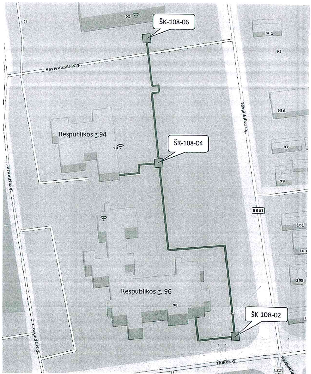
Šilumos tinklų nuo ŠK-108-02 iki ŠK-108-06 su atšakomis Rokiškyje situacijos schema
