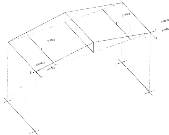
2 pav. Maksimaliai leistinos scenos konstrukcijos apkrovos
