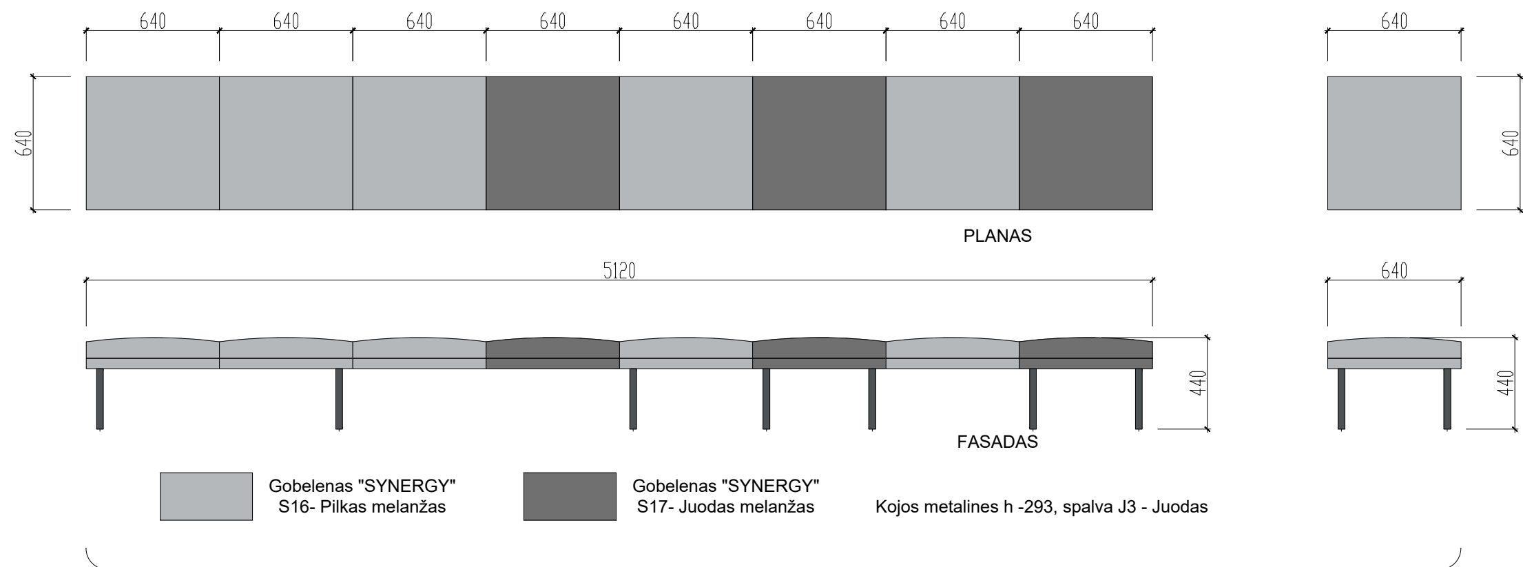
F1 Minkštasuolis 5120x640, h-450mm, be atlošo, be porankių pagal kolekciją "Archipelago" "Narbutas"
