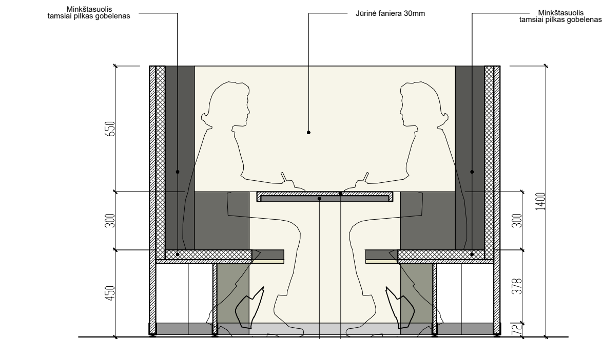
PJŪVIS A-A
