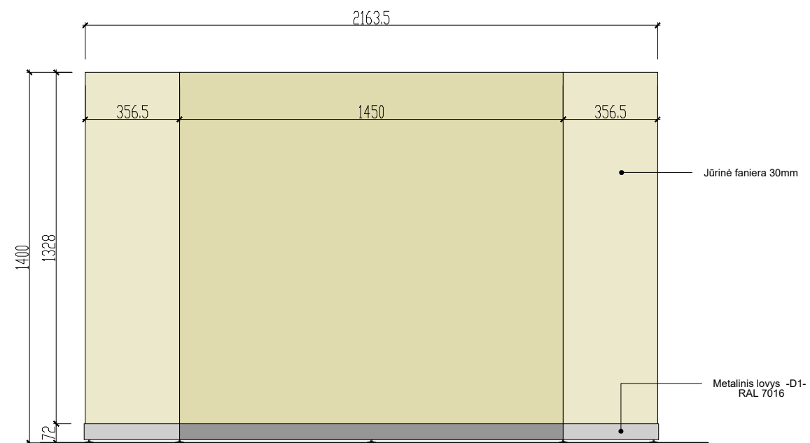
PJŪVIS D-D
