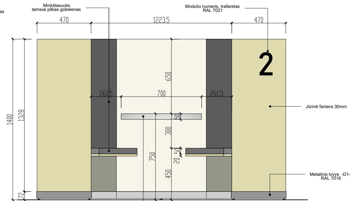
PJŪVIS C-C
