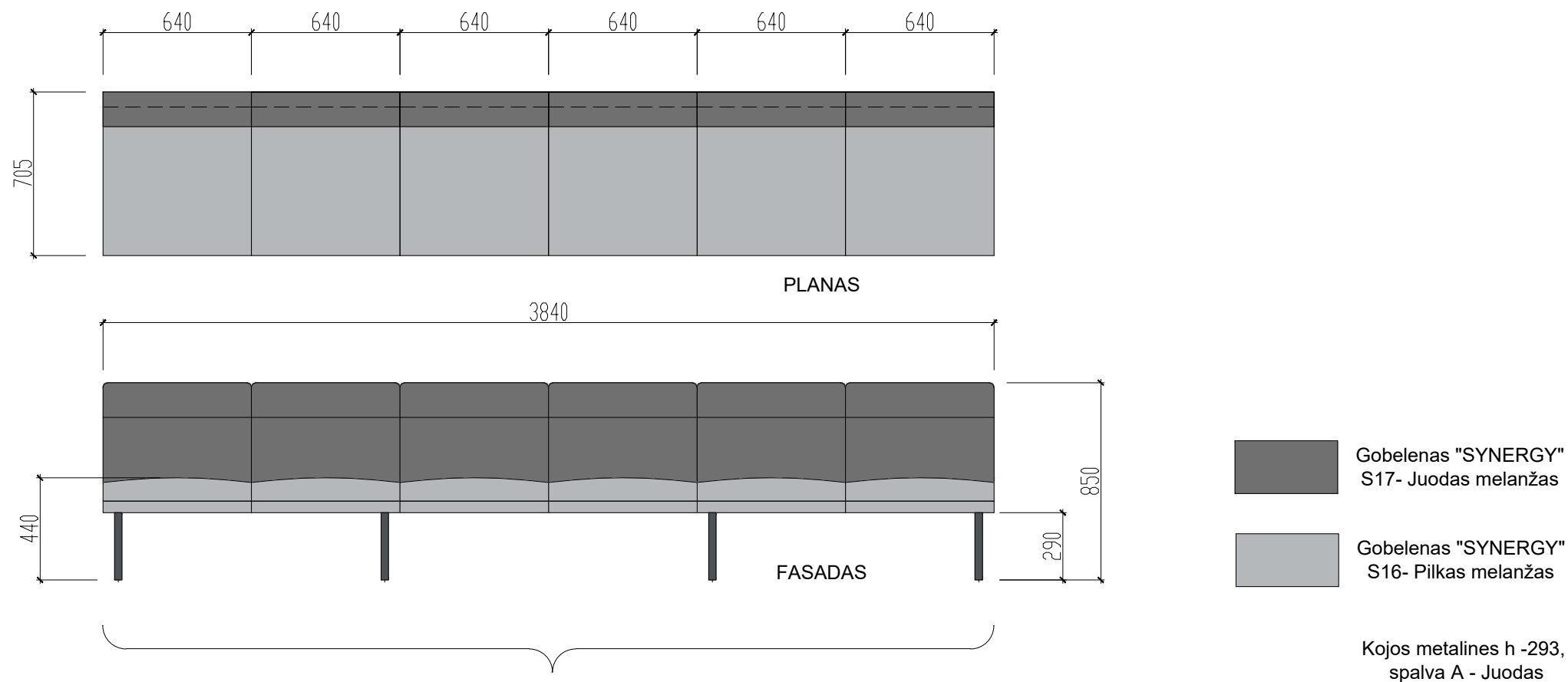
F2 Minkštasuolis 3840x705, h-450/850mm, su atlošu, be porankių pagal kolekciją "Archipelago" "Narbutas"
