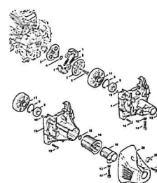
Sankaba, sankabos korpusas
