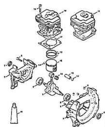
Karteris, cilindras
