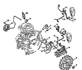
Uždegimo sistema
