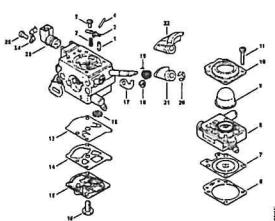
Karbiuratorius WTF-7, WTF-12
