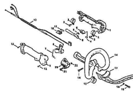
Kilpinė rankena
