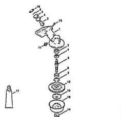
Reduktorius FS 460 RC
