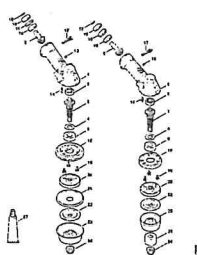
Reduktorius FS 460 C
